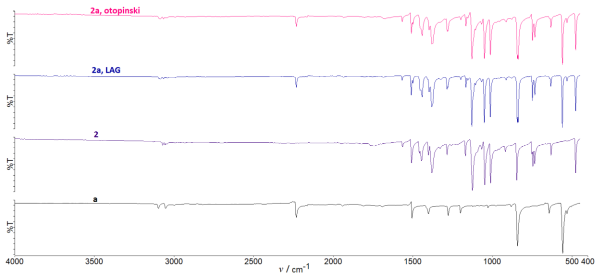
Slika D38. Usporedba IR spektara kokristala [\text{CdI}_2(\text{Br-pz})_2][1,4\text{-DCB}] ( 2a ) dobivenog mehanokemijskom sintezom i otopinskom sintezom s polaznim spojevima: [\text{CdI}_2(\text{Br-pz})_2]_n ( 2 ) i 1,4-dicijanobenzenom ( a ).
