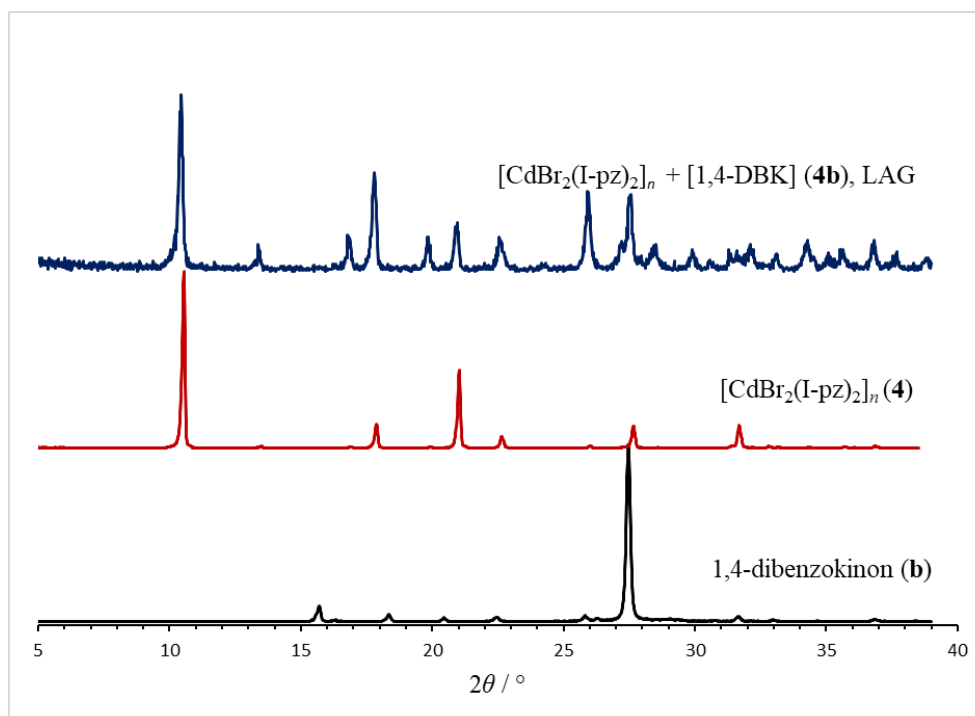
Slika D19. Usporedba difraktograma praškastih uzoraka reaktanata [\text{CdBr}_2(\text{I-pz})_2]_n ( 4 ) i 1,4-benzokininona ( b ) i produkta mljevenja potpomognutog kapljevnom ( 4b ).
