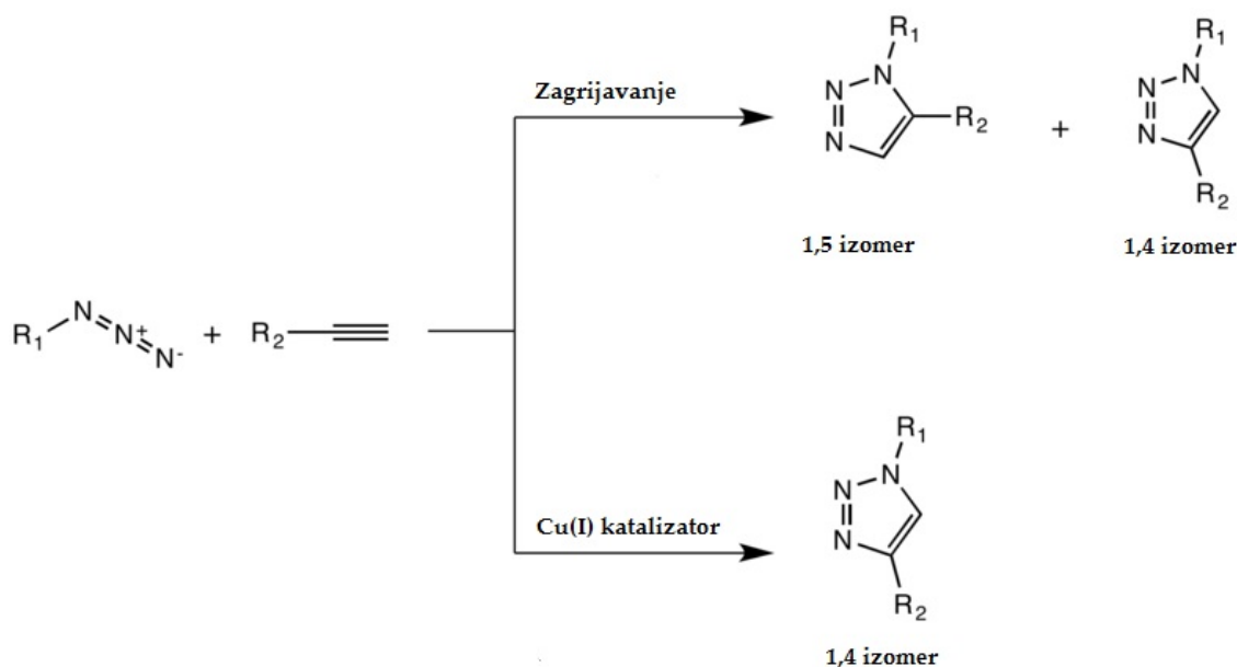
Shema 1. Cikloadicija azida na alkine
