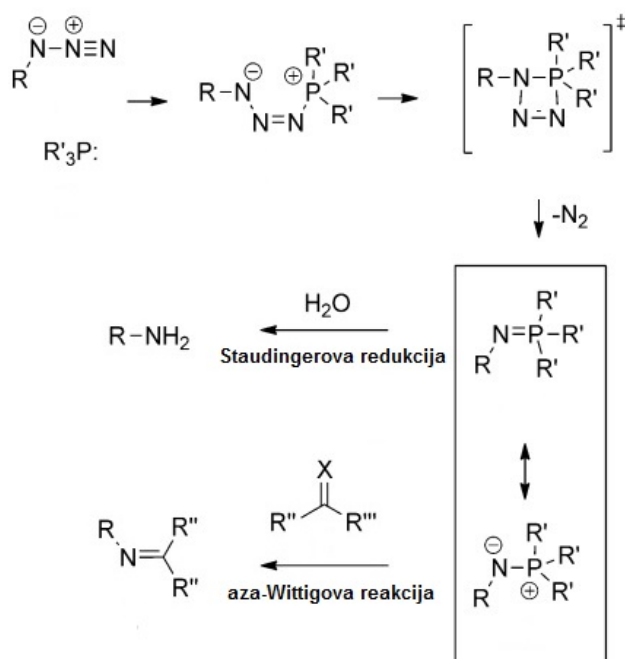
Shema 2. Mehanizam Staudingerove redukcije
