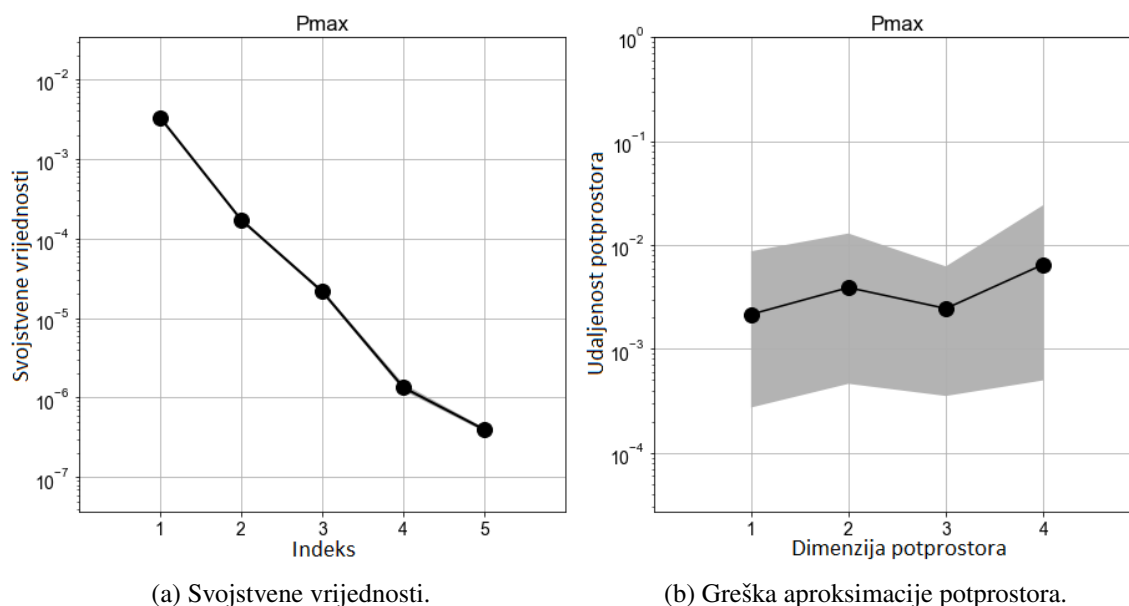
Slika 3.1: Na lijevoj slici vidimo svojstvene vrijednosti matrice \hat{C} . Desna slika prikazuje procjenu greške aproksimacije potprostora.
