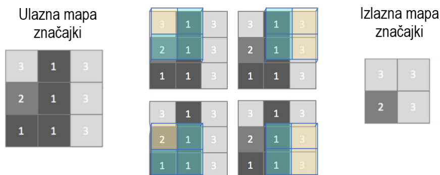
Slika 5.7: Sažimanje maksimalnom vrijednošću. Izlazna mapa značajki predstavlja vrijednost nakon odabira maksimalnih vrijednosti. Maksimalne vrijednosti u svakom 2 \times 2 okviru označene su žutom bojom. Vrijednosti parametara su F = 2 i S = 1 . Izvor [20].
