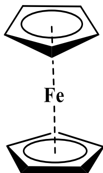
Slika 1. Ferocen (Fc).
