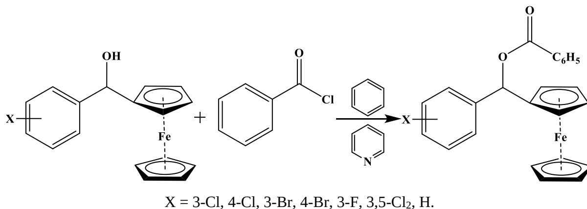
Shema D9. Priprava različito supstituiranih fenilferocenilmetil-benzoata.
