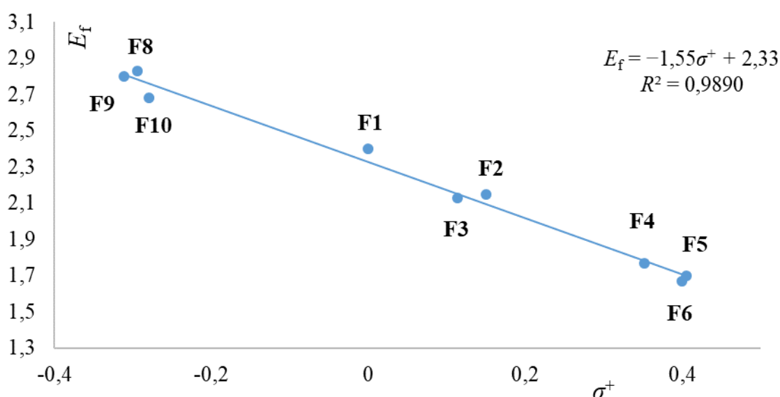
Slika 22. Korelacija parametra elektrofugalnosti E_f fenilferocenilmetilnih elektrofuga ( F1 – F6 i F8 – F10 ) i Hammett-Brownova parametra \sigma^+ .
