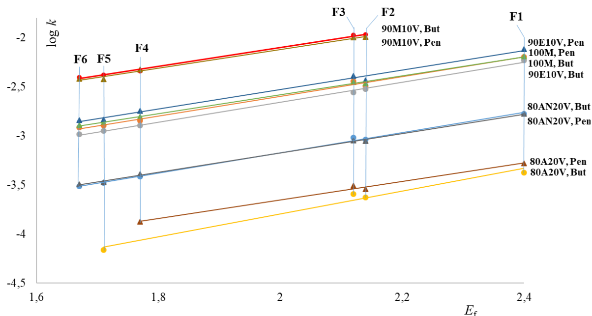
Slika 19. Ovisnost \log k o E_f za solvolizu supstituiranih fenilferocenilmetilnih butanoata i pentanoata u različitim otapalima. 106 Butanoat = \text{CH}_3\text{CH}_2\text{CH}_2\text{COO}^- , Pentanoat = \text{CH}_3\text{CH}_2\text{CH}_2\text{CH}_2\text{COO}^- . Smjesa otapala je prikazana kao volumni udio otapala u smjesi; A = aceton, AN = acetonitril, E = etanol, M = metanol i V = voda.
