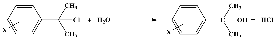
Shema 6. Solvoliza supstituiranih \alpha -kumil-klorida.
