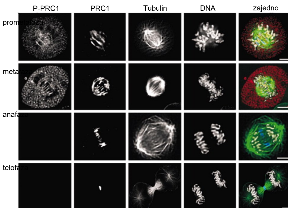
Slika 2.7. Lokalizacija proteina regulatora citokineze 1. P-PRC1 je fosforilirani monomer kojeg ne mogu defosforilirati fosfataze, a PRC1 je funkcionalni protein. Skala je 1 \mu m. Preuzeto i obrađeno prema ref. 18
