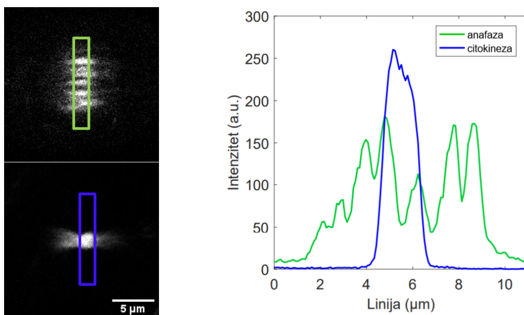
Slika 4.10. Usporedba profila intenziteta signala PRC1-GFP u anafazi (zeleno) i telofazi/citokinezi (plavo). Skala je na svim slikama 5 \mu\text{m} . Profil je širok 12 piksela.
