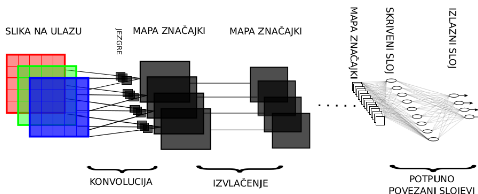
Slika 2.6: Uobičajena struktura konvolucijske neuronske mreže [16]
