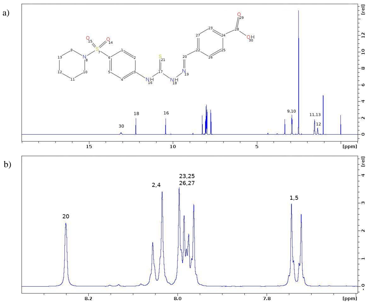
Slika 46. Spektar 1 H NMR tiosemikarbazona-10: a) cijeli spektar, b) uvećani dio spektra u području od 7,6 ppm do 8,4 ppm.
