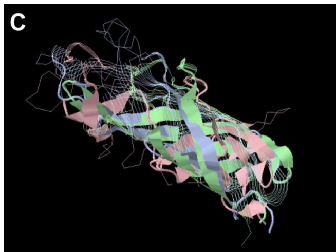
Slika 2. Domene II i III proteina EF-Tu koje tvore dvije hidrofobne bačve u poklapanju s transmembranskim regijama proteina OmpW i OprF. Preuzeto i prilagođeno iz N'Diaye i sur., 2019.
