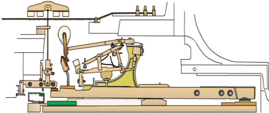
Slika 1.7: Prikaz kako udarna poluga sklizne s rollice.
