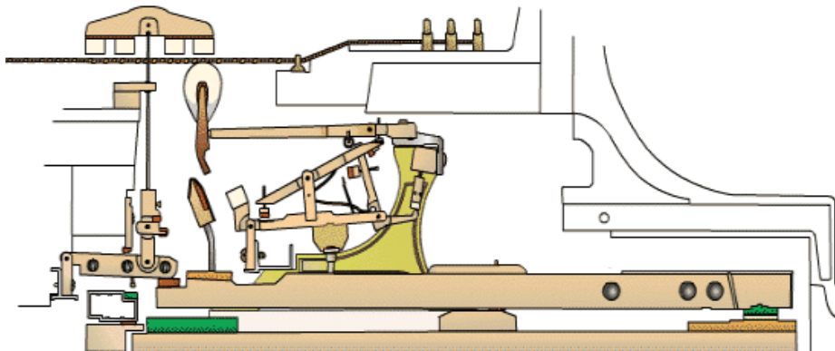
Slika 1.6: Prikaz kontakta batića i žice.
