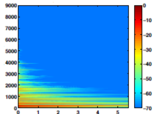
Slika 3.4: Spektrogram - egzaktno Frekvencije (Hz) kroz vrijeme (s).
