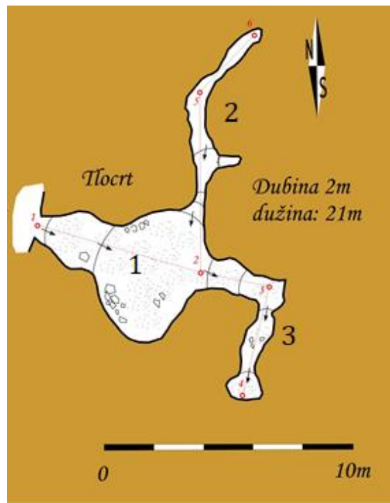
Slika 10. Tlocrt Sedrene špilje kod stola (autor nacрта: J. Radaljac, modificirano) s označenim dijelovima špilje (1 – prvi dio, 2 – drugi dio, 3 – treći dio), izvor: Državni speleološki katastar (URL 5).
