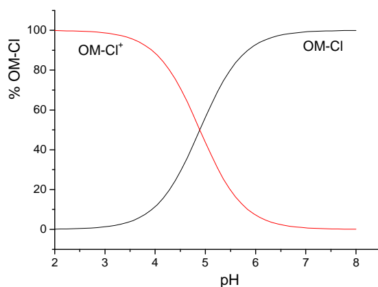
Slika 38. Distribucijski dijagram otopine spoja OM-Cl u miješanom otapalu MeOH/H 2 O pri (25,0 \pm 0,1) \text{ }^\circ\text{C} ; V(\text{MeOH})/V(\text{H}_2\text{O}) = 1:1 , I_c = 0,05 \text{ mol dm}^{-3} (TBAClO 4 ).
