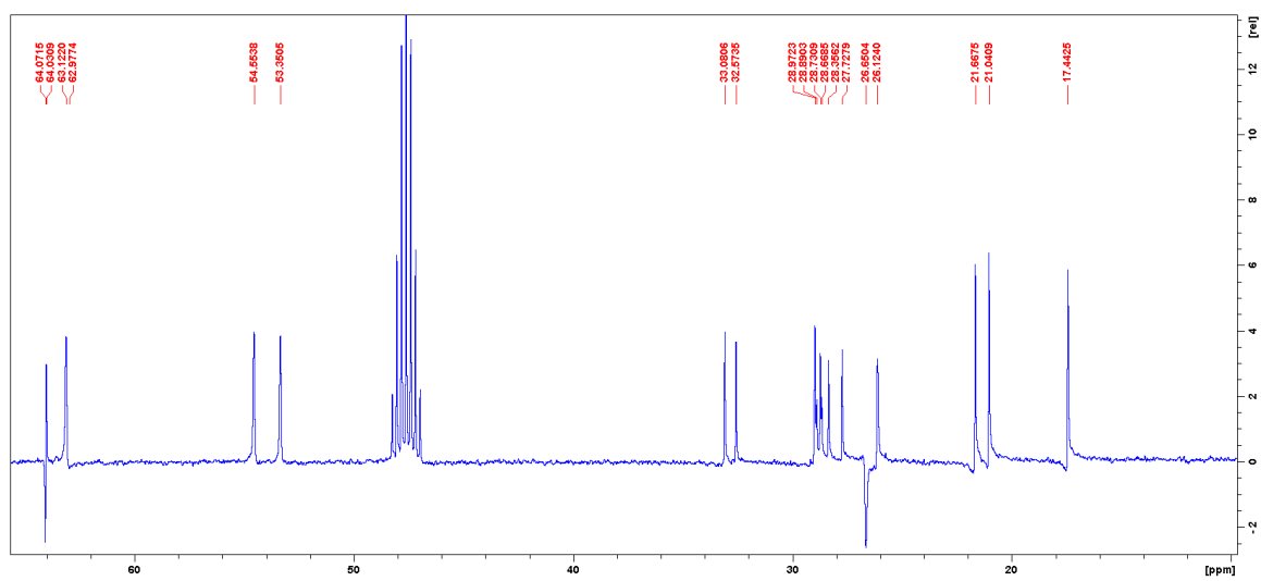
Slika D34 ^{13}\text{C} NMR spektar spoja 20
