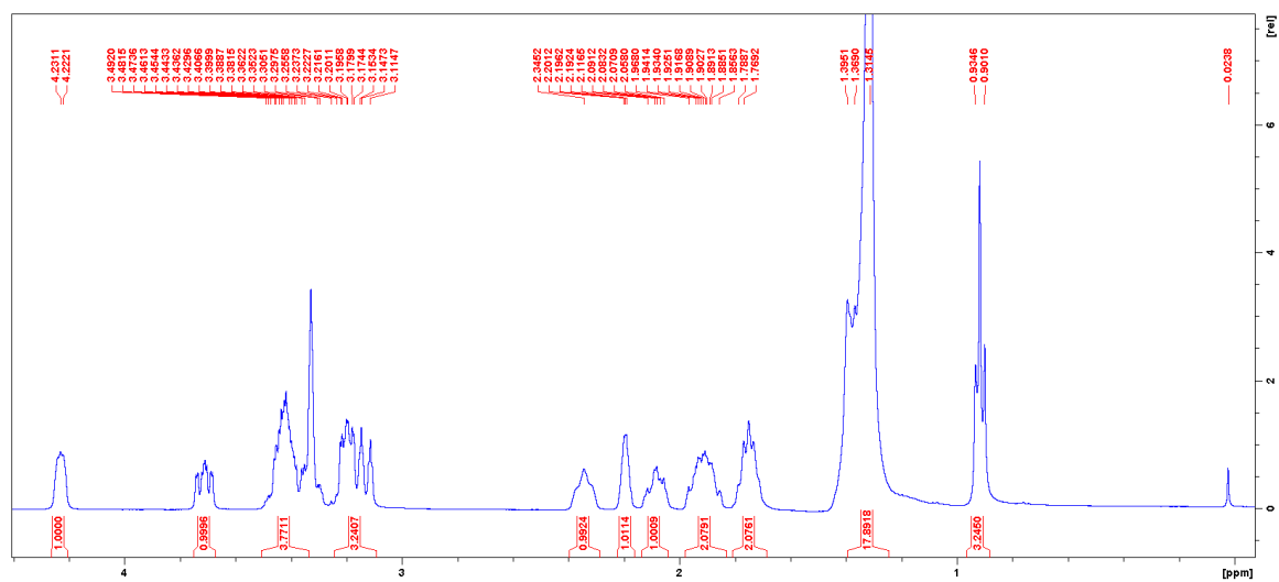
Slika D17. ^1\text{H} NMR spektar spoja 12
