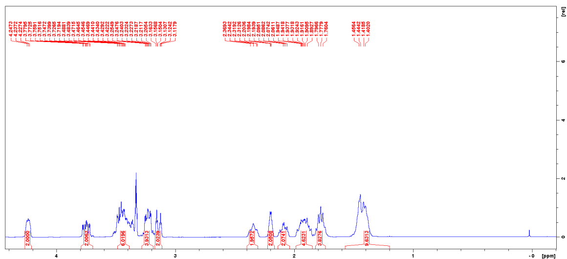
Slika D33. ^1\text{H} NMR spektar spoja 20
