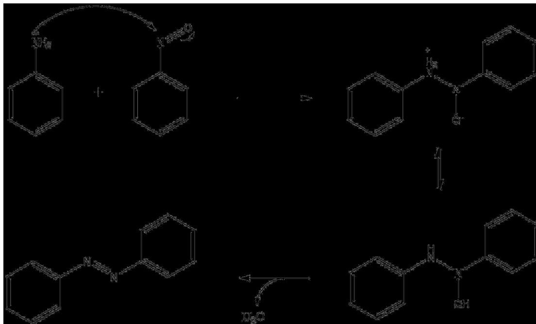
Slika 12. Mehanizam Millsove reakcije
