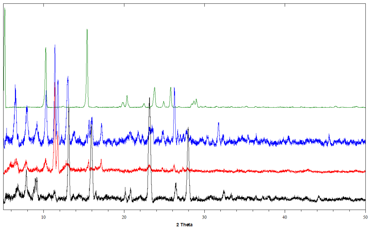
Slika D38. Usporedba difraktograma praha kompleksnog spoja [Cu(H 2 T)] 2 (crno) s difraktogramima praha liganda (zeleno), kompleksnog spoja dobivenog sintezom na ultrazvučnoj kupelji (crveno) i kompleksnog spoja dobivenog mehanokemijskom sintezom (plavo)
