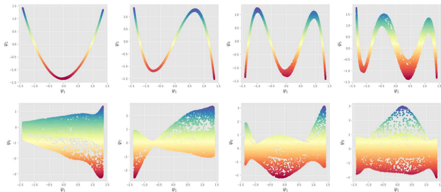
Slika 3.9: Prikaz švicarske role s pomoću različitih difuzijskih koordinata koje su označene na koordinatnim osima. U prvom slučaju za parametre t = 1 , \varepsilon = 2 , k = 100 , \alpha = 0 , a u drugom za t = 1 , \varepsilon = 25 , k = 10 , \alpha = 0 . Primijetimo kako za prvu kombinaciju parametara npr. šesta difuzijska koordinata daje najbolju realizaciju odmotane švicarske role. Za drugu kombinaciju to se postiže koristeći četvrtu ili petu difuzijsku koordinatu.
