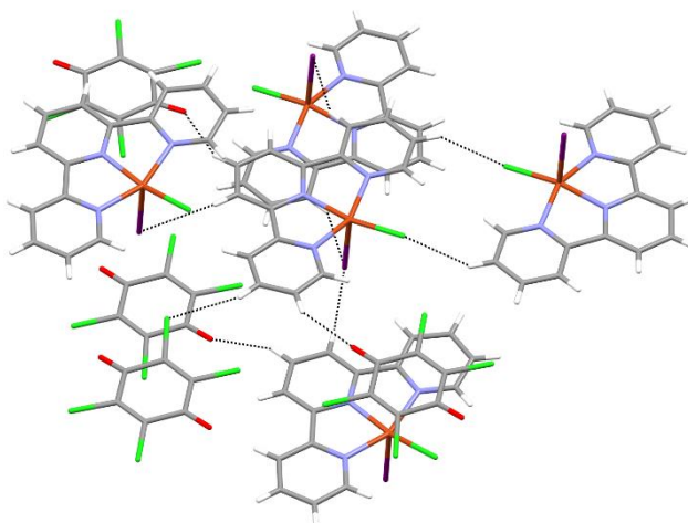
Slika 132. Vodikove veze (isprekidane crte) i \pi -interakcije prisutne u spoju [Cu(terpy)ICl][C 6 O 2 Cl 4 ] ( 2t ).
