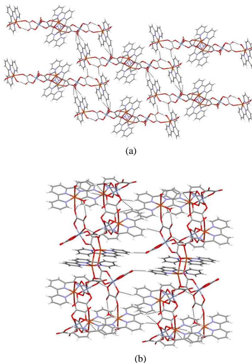
Slika 66. Prikaz vodikovih veza (isprekidane crte) između: (a) susjednih kationa u ravnini ac i (b) susjednih kationa i aniona u ravnini bc s \pi -interakcijama između aromatskih prstenova terpiridina u kristalnoj strukturi spoja [\text{Cr}_2\text{Cu}_4(\text{H}_2\text{O})_4(\text{terpy})_4(\text{C}_2\text{O}_4)_6][\text{Cr}_2\text{Cu}_2(\text{terpy})_2(\text{C}_2\text{O}_4)_6] \cdot 10\text{H}_2\text{O} ( 17o )
