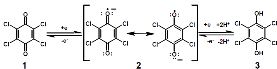
Slika 19. Tri odabrana tipa planarnih konjugiranih prstenova: kinoidni (tetraklorkinon, 1), semikinonski (tetraklorsemikinon, 2) i aromatski (tetraklorhidrokinon, 3). 57
