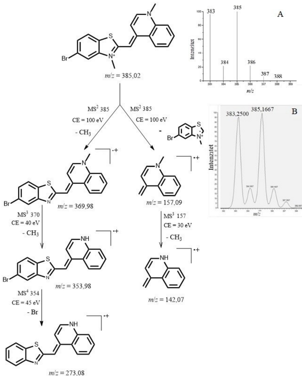
Shema 2. Prikaz puta fragmentiranja molekuskog iona (signal m/z = 385 ) prema spektrima ESI MS za marker 1 (otopljen u otopini amonijevog acetata, acetonitrila i vode, c = 38,65 \mu\text{mol L}^{-1} ) s umetkom A na kojem je prikazan teoretski spektar markera 1 i umetkom B na kojem je prikazan uvećani i razvučeni spektar markera 1 za signal m/z = 385 , izolacijska širina = \pm 1 (CE = kolizijska energija).
