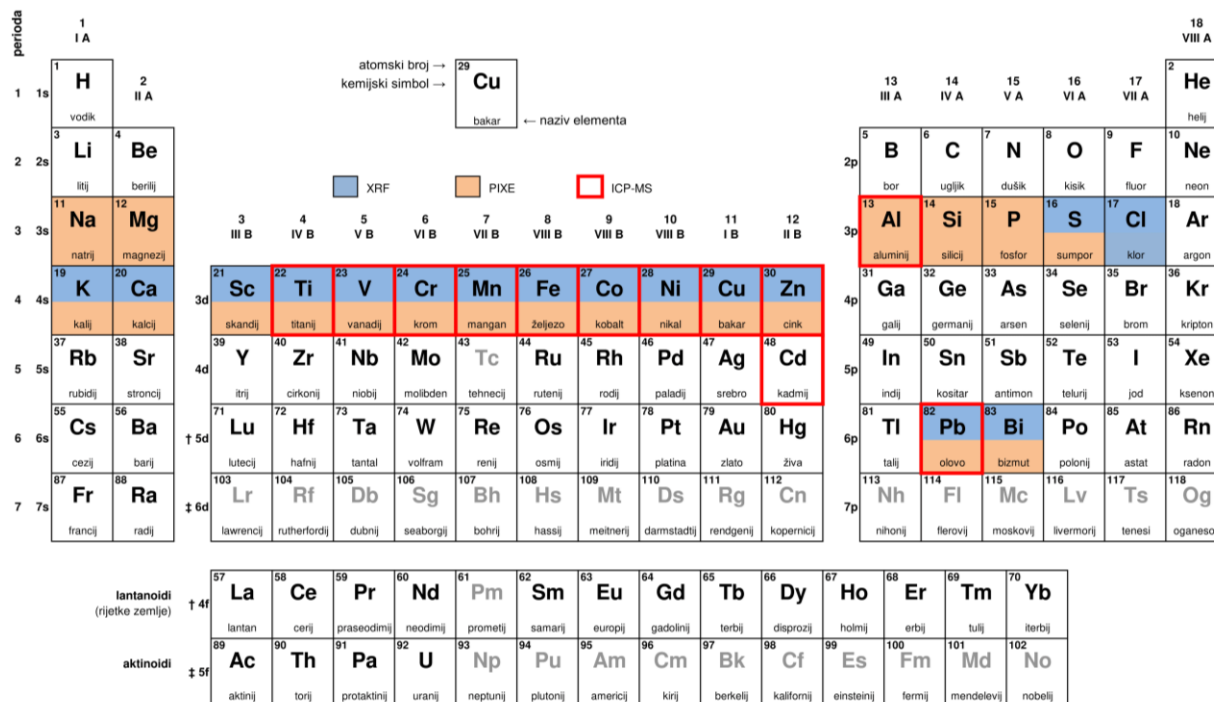
Slika 2.13. Periodni sustav elemenata s označenim elementima čije su koncentracije u ovom radu dobivene metodama XRF, PIXE i ICP-MS. [170], nazivi elemenata prema [171].
