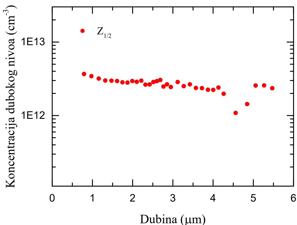
Slika 36: Profil dubokog nivoa uzorka ozračenog najvećom dozom (100Gy) izračunan uporabom DLTS tehnike na 315K. Korišten je vremenski prozor koji odgovara emisiji 50\text{s}^{-1} . U obzir je uzet lambda efekt.
