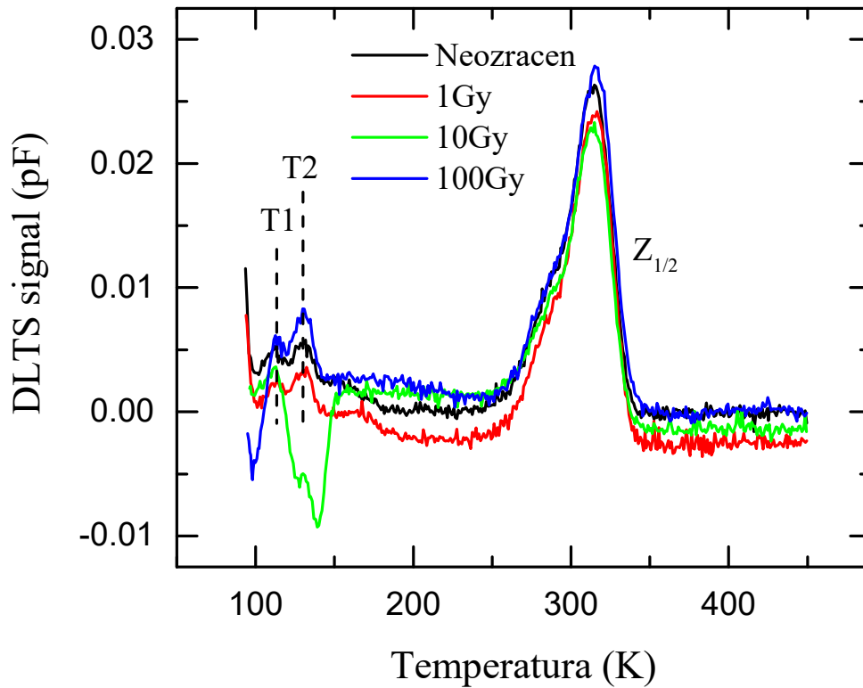
Slika 35: DLTS spektar uzoraka ozračenih u realnim uvjetima. Korišten je reverzni napon V_R = -10V i napon pulsa V_P = -0.1V trajanja t_p = 10ms . Prikazan je vremenski prozor 50s^{-1} .
