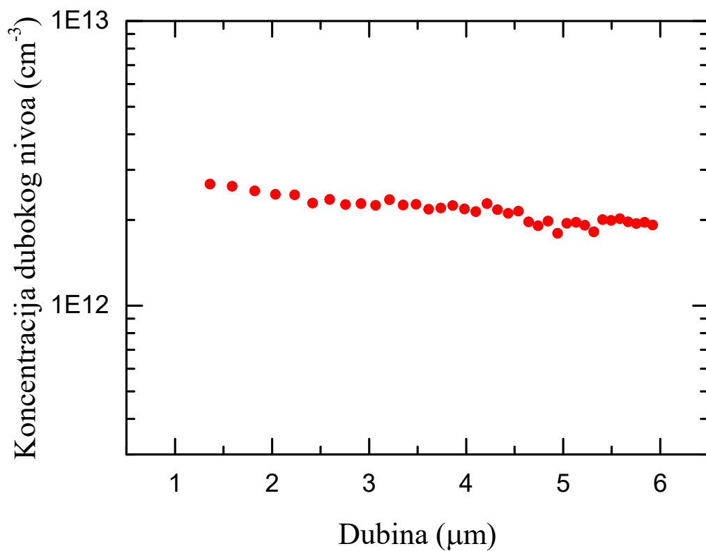
Slika 20: Dubinski profil dubokog nivoa neozračenog B1 uzorka na 315K koji odgovara vakanciji ugljika V_C(2-/0) . Korišten je vremenski prozor koji odgovara emisiji 50s^{-1} . U obzir je uzet lambda efekt.
