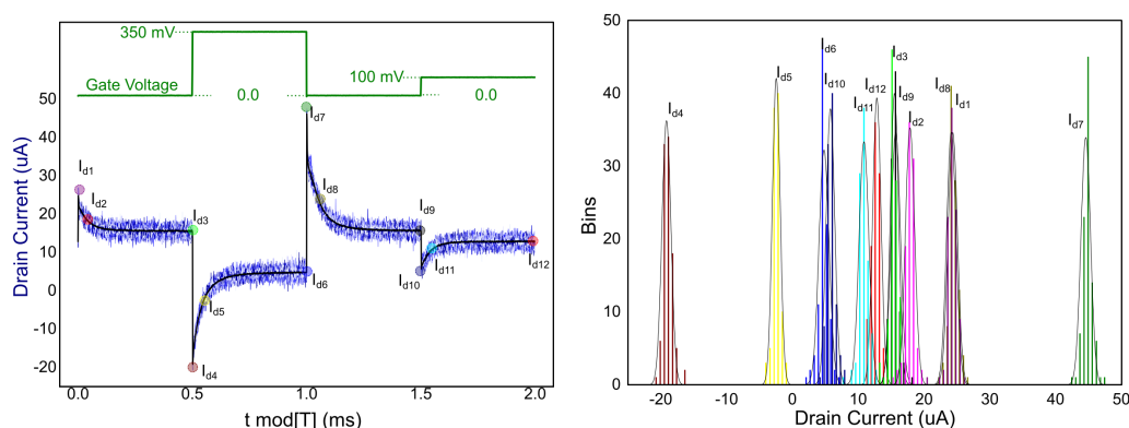
Slika 7.3: a) Uzorak signala odvodne struje u trajanju od 2-ms za jedno mjerenje 0.1 M KCl aq od 200-ms. b) Statistička raspodjela 12 karakterističnih vrijednosti uzetih iz signala odvodne struje jednog 200-ms mjerenja 0.1 M KCl aq . Slika je uzeta iz [28].
