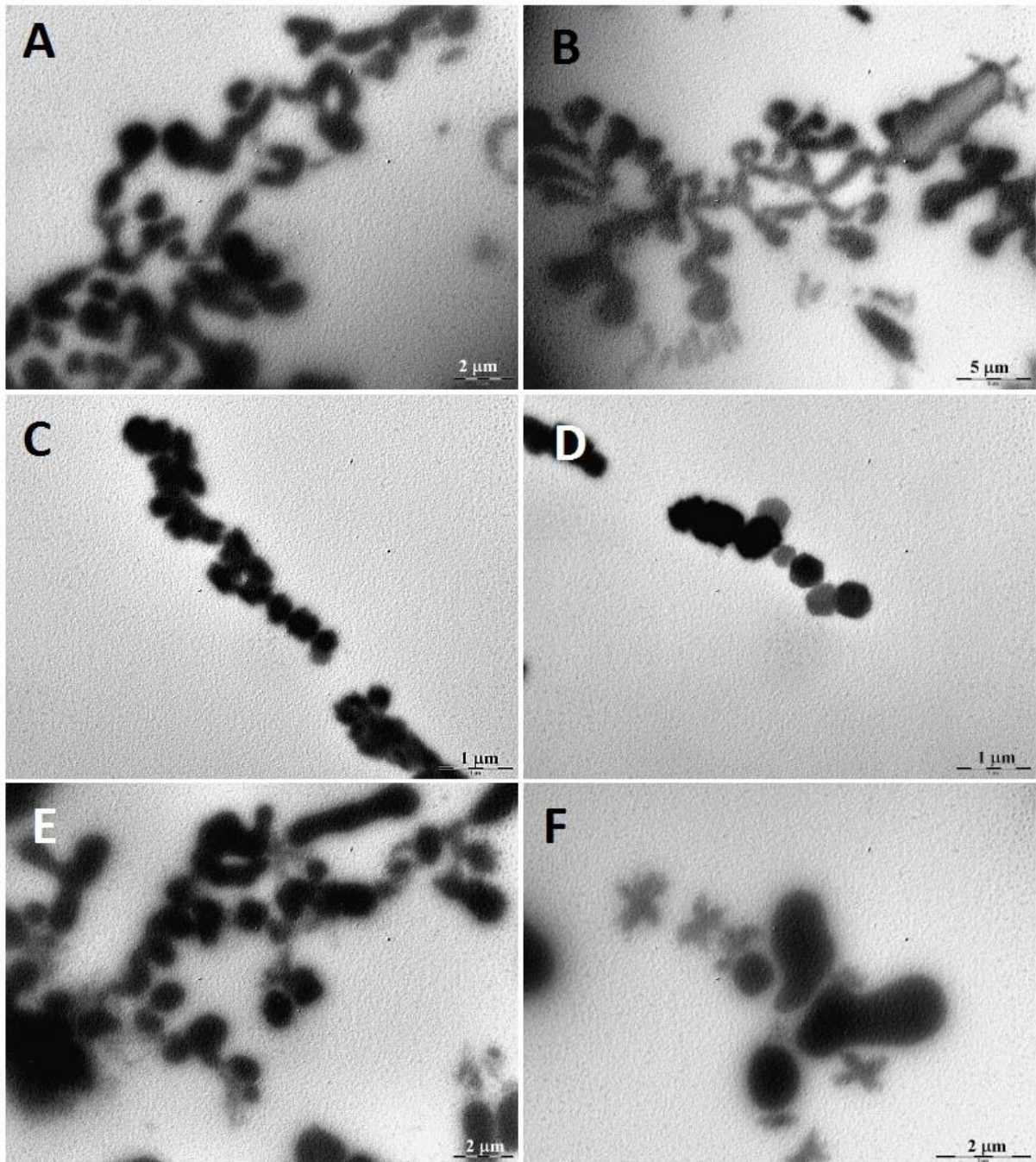
Slika 48. TEM mikrografije nanočestica srebra promjera 60 nm (Ag60 LMNB) dispergiranih u umjetnoj morskoj vodi saliniteta 15 (ASW 15) s dodatkom 10 \text{ mg mL}^{-1} Tweena 80. Svaka od slika (A-F) predstavlja mikrografiju istog uzorka. Koncentracija nanočestica bila je 5 \text{ } \mu\text{g mL}^{-1} . Nanočestice su dispergirane u mediju (ASW) 48 sati pri sobnoj temperaturi.
