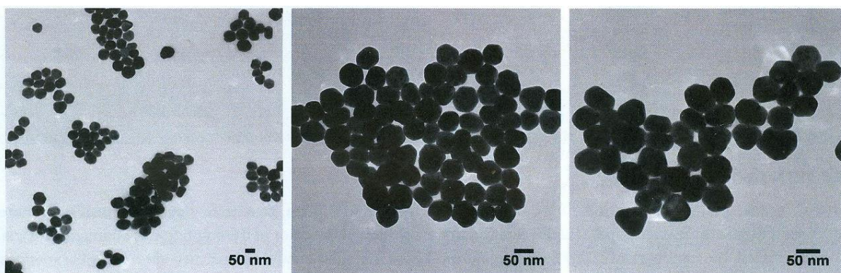
Slika 3. TEM mikrografije komercijalnih nanočestica srebra omotanih citratom (kupljene od tvrtke Nanocomposix, San Diego, CA) prosječne veličine (promjera) 60 nm.
