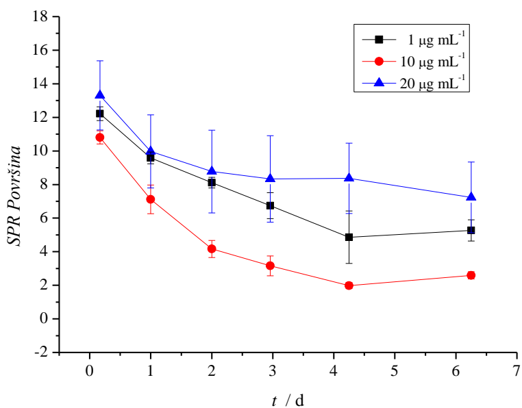
Slika 38. Promjene SPR površine pika nanočestica srebra promjera 60 nm (Ag60 NC, masene koncentracije 5 µg mL -1 ) kojima je dodan supernatant celomske tekućine ježinca P. lividus različitog sadržaja proteina (1 – 20 µg mL -1 ) u ultračistoj vodi tijekom 6 dana pri sobnoj temperaturi.
