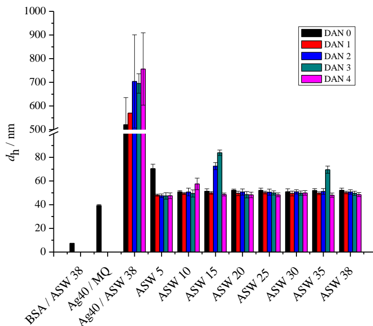
Slika 23. Promjena hidrodinamičkih promjera ( d_h ) s vremenom za nanočestica srebra ( 5 \mu\text{g mL}^{-1} ) nominalne veličine 40 nm. Nanočesticama je dodan BSA ( 100 \mu\text{M} ) u ultračistoj (MQ) i umjetnoj morskoj vodi (ASW) različitih saliniteta (5-38). Mjerenja su izvedena pri sobnoj temperaturi.
