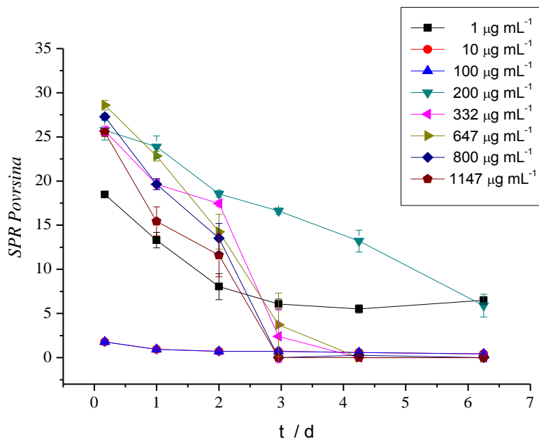
Slika 35. Promjene SPR površine pika nanočestica srebra promjera 60 nm (Ag60 NC, masene koncentracije 5 µg mL -1 ) kojima je dodan supernatant hemolimfe dagnje M. galloprovincialis različitog sadržaja proteina (1 – 1147 µg mL -1 ) u ultračistoj vodi tijekom 6 dana pri sobnoj temperaturi.
