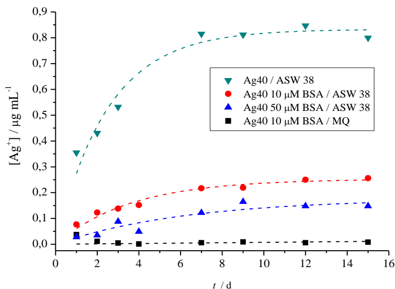
Slika 34. Koncentracija otopljenog srebra poteklog od nanočestica srebra promjera 40 nm početne koncentracije 1 µg mL -1 s dodatkom 10 i 50 µM BSA u umjetnoj morskoj vodi saliniteta 38, bez BSA i u ultračistoj vodi (MQ). Mjerni podaci modelirani su Box Lucas I funkcijom u programu OriginPro, a vrijednosti dobivenih krivulja prikazane su u Tablici 13. Eksperiment i mjerenja provedeni su pri sobnoj temperaturi.
