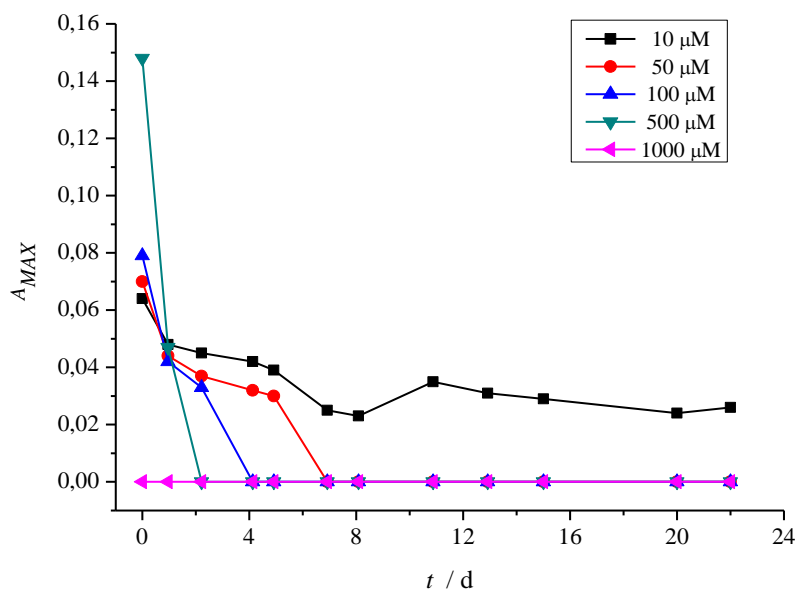
Slika 27. Maksimumi apsorbancije, A_{MAX} , za disperzije nanočestica srebra (Ag40) masene koncentracije 0,5 \mu\text{g mL}^{-1} uz dodatak različitih koncentracija BSA (10 – 1000 \mu\text{M} ) u umjetnoj morskoj vodi saliniteta 38. Eksperimenti i mjerenja izvedeni su pri sobnoj temperaturi.
