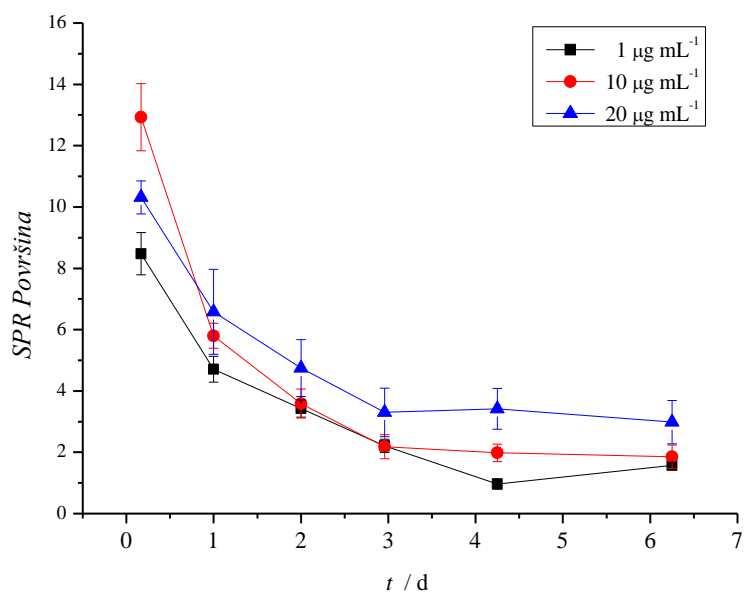
Slika 39. Promjene SPR površine pika nanočestica srebra promjera 60 nm (Ag60 NC, masene koncentracije 5 µg mL -1 ) kojima je dodan supernatant celomske tekućine ježinca P. lividus različitog sadržaja proteina (1 – 20 µg mL -1 ) u umjetnoj morskoj vodi saliniteteta 15 tijekom dana pri sobnoj temperaturi.
