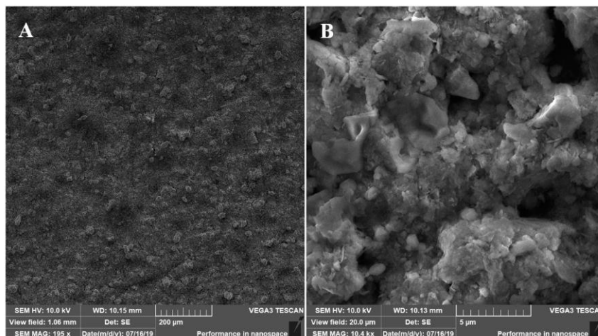
Slika 13. SEM mikrografija prirodnog sedimenta iz Limskog kanala (NS), pod povećanjem od A) 195 puta i B) 10400 puta.
