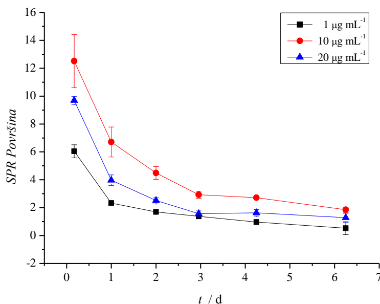
Slika 40. Promjene SPR površine pika nanočestica srebra promjera 60 nm (Ag60 NC, masene koncentracije 5 \mu\text{g mL}^{-1} ) kojima je dodan supernatant celomske tekućine ježinca P. lividus različitog sadržaja proteina ( 1 - 20 \mu\text{g mL}^{-1} ) u umjetnoj morskoj vodi saliniteteta 38 tijekom dana pri sobnoj temperaturi.
