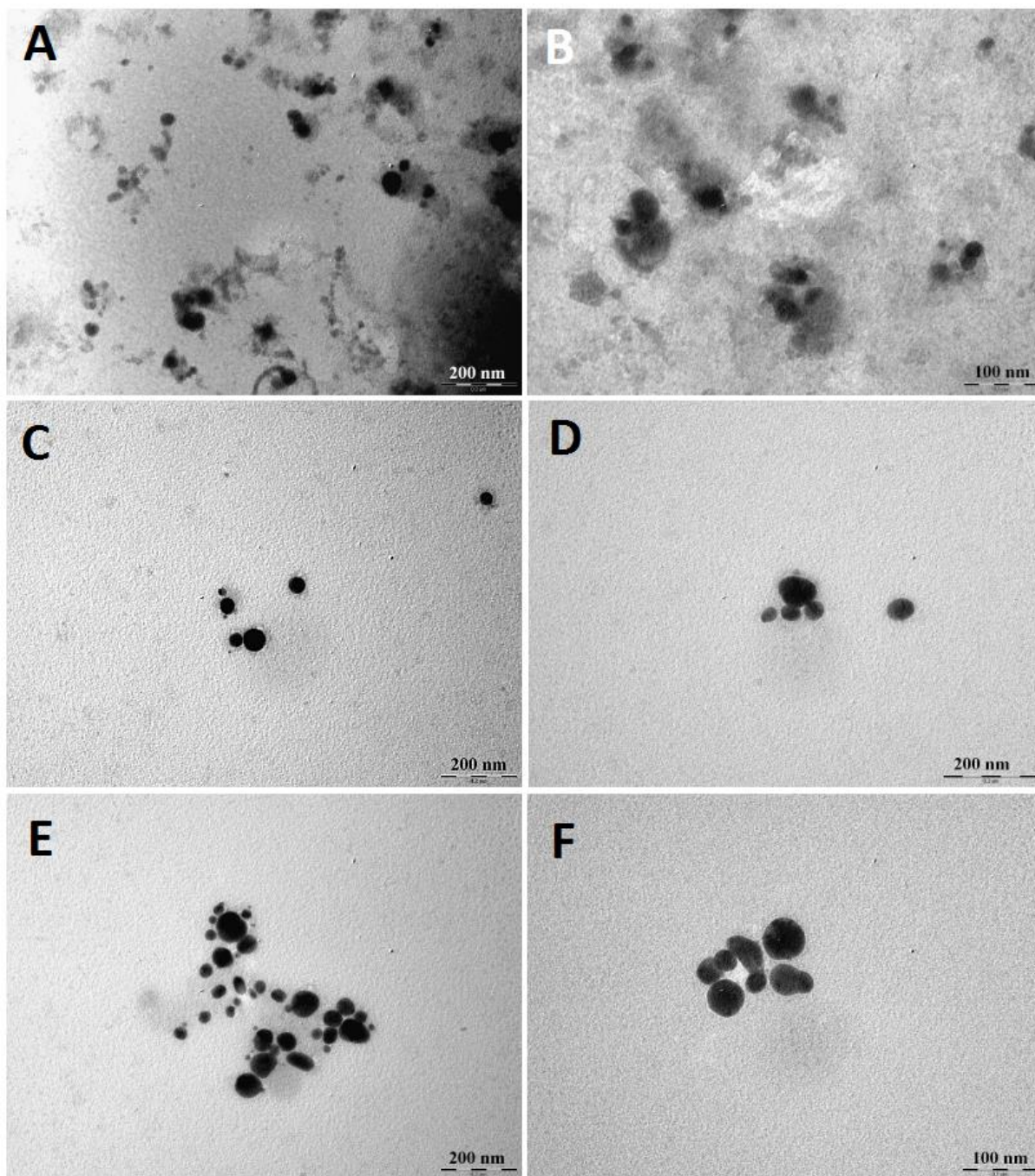
Slika 49. TEM mikrografije nanočestica srebra promjera 60 nm (Ag60 LMNB) dispergiranih u filtriranoj prirodnoj morskoj vodi saliniteta 15 (FSW 15) s dodatkom 10 \text{ mg mL}^{-1} Tweena 80. Svaka od slika (A-F) predstavlja mikrografiju istog uzorka. Koncentracija nanočestica bila je 5 \text{ } \mu\text{g mL}^{-1} . Nanočestice su odstajale u mediju 48 sati, a eksperiment i snimanje izvršeni su pri sobnoj temperaturi.
