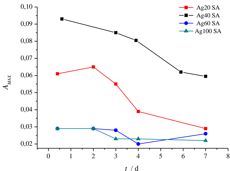
Slika 18. Apsorbancijski maksimumi, A_{MAX} , u ovisnosti o vremenu za disperzije nanočestica srebra različite veličine; 20, 40, 60 i 100 nm (Ag20 SA, Ag40 SA, Ag60 SA i Ag100 SA), masene koncentracije 1 \mu\text{g mL}^{-1} i koncentracije BSA 100 \mu\text{M} u umjetnoj morskoj vodi saliniteta 38. Eksperiment i mjerenja vršeni su pri sobnoj temperaturi.
