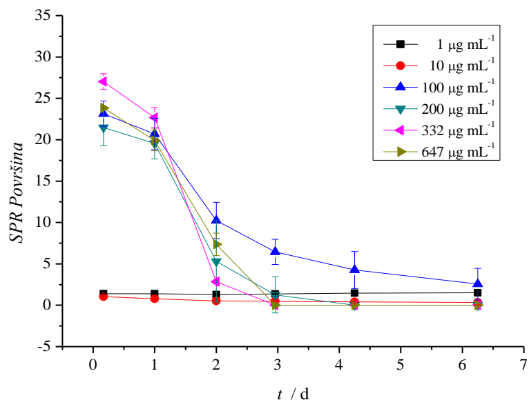
Slika 36. Promjene SPR površine pika nanočestica srebra promjera 60 nm (Ag60 NC, masene koncentracije 5 µg mL -1 ) kojima je dodan supernatant hemolimfe dagnje M. galloprovincialis različitog sadržaja proteina (1 – 647 µg mL -1 ) u umjetnoj morskoj vodi saliniteta 15 tijekom 6 dana pri sobnoj temperaturi.
