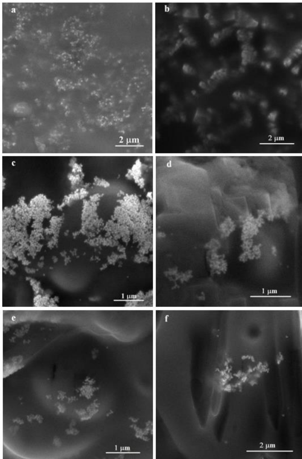
Slika 47. SEM mikrografije nanočestica srebra ( \text{Ag}_{60} NC, 5 \mu\text{g mL}^{-1} ) s dodatkom Tweena ( 1 \text{ mg mL}^{-1} ) u a) umjetnoj morskoj vodi saliniteta 15, b) umjetnoj morskoj vodi saliniteta 35, c) u filtriranoj prirodnoj morskoj vodi saliniteta 15, d) filtriranoj prirodnoj morskoj vodi saliniteta 35, e) prirodnoj nefiltriranoj morskoj vodi saliniteta 15 i f) prirodnoj nefiltriranoj morskoj vodi saliniteta 35. Eksperiment i mjerenja provedeni su pri sobnoj temperaturi, a nanočestice su u medijima bile 48 sati.
