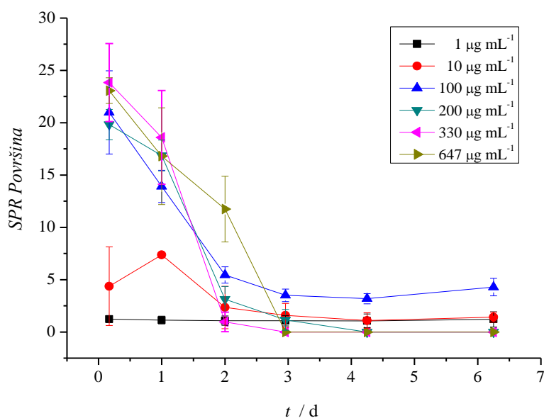
Slika 37. Promjene SPR površine pika nanočestica srebra promjera 60 nm (Ag60 NC, masene koncentracije 5 \mu\text{g mL}^{-1} ) kojima je dodan supernatant hemolimfe dagnje M. galloprovincialis različitog sadržaja proteina ( 1 - 647 \mu\text{g mL}^{-1} ) u umjetnoj morskoj vodi saliniteta 38 tijekom 6 dana pri sobnoj temperaturi.
