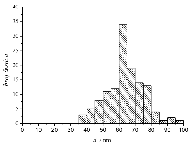
Slika 10. Histogram promjera ( d ) nanočestica srebra sintetiziranih u Laboratoriju za morską nanotehnologiju i biotehnologiju (Ag60 LMNB). Promjeri su dobiveni analizom mikrografije sa Slike 9 u programu ImageJ.
