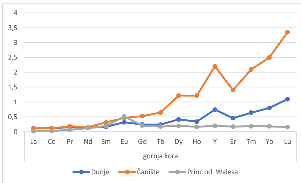
Slika 21. Graf vrijednosti REE-ova normaliziranih na gornju koru
