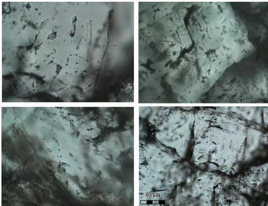
Slika 18. Primarne fluidne inkluzije uzorka sa lokaliteta Čanište
