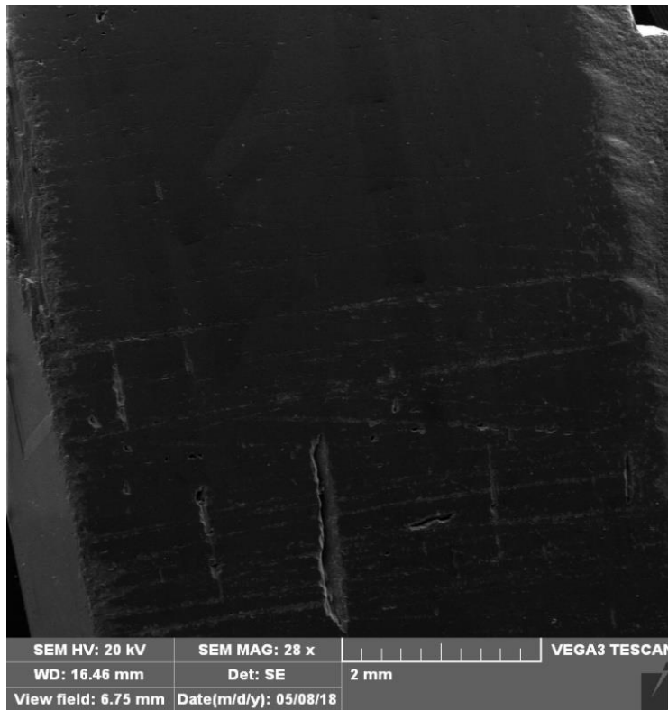
Slika 12. BSE slika plohe (101)
