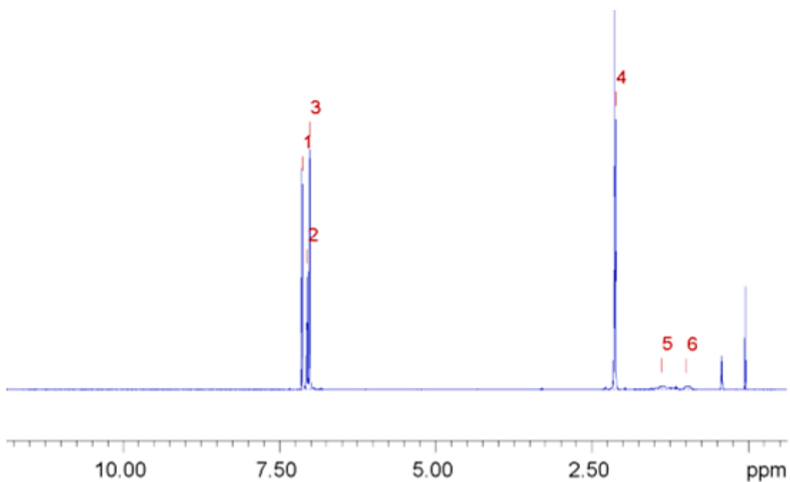
Slika D10a. Reprezentativni spektar ^1\text{H} NMR uzorka asfaltena VO1 ( \gamma = 0,03 \text{ g L}^{-1} ) izoliranog iz vakuumskog ostatka nafte 2 snimljen u toluenu- d_8 pri 400 MHz i 25°C
