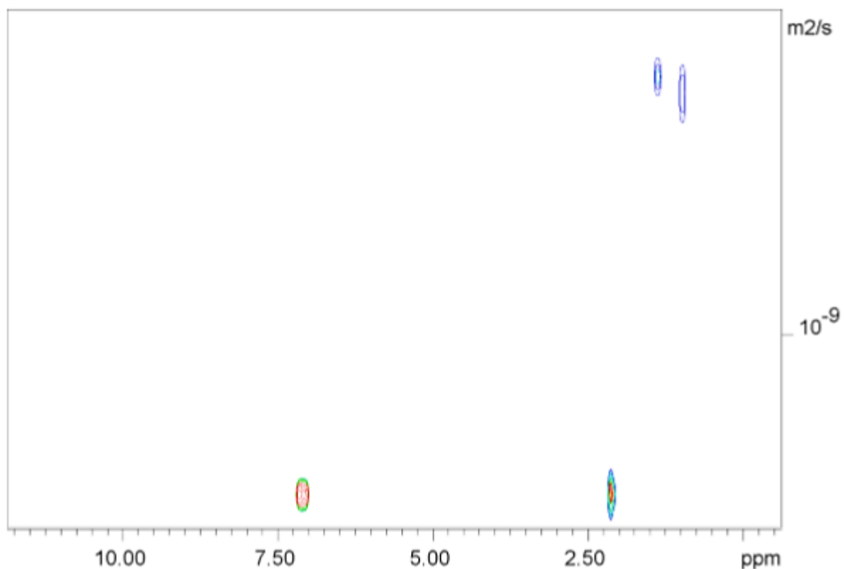
Slika D10b. Reprezentativni spektar DOSY NMR uzorka asfaltena VO1 ( \gamma = 0,03 \text{ g L}^{-1} ) izoliranog iz vakuumskog ostatka nafte 2 snimljen u toluenu- d_8 pri 400 MHz i 25°C.
