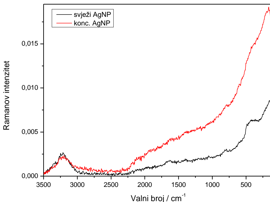
Slika 9. Ramanov spektar svježeg pripravljenog i koncentriranog koloida srebra.
