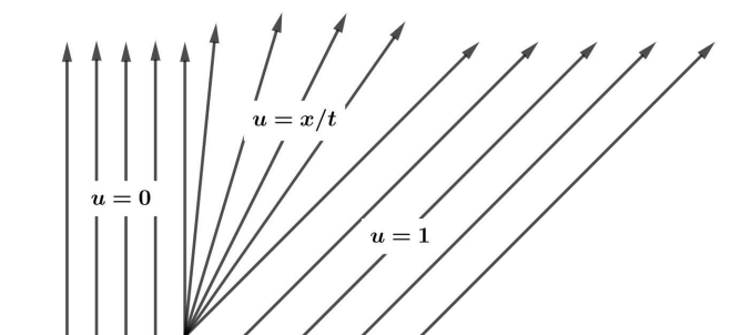
Slika 2.3: Val refrakcije
