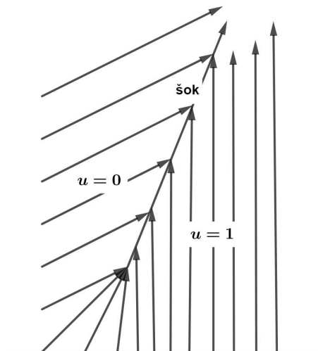
Slika 2.1: Nastanak šoka
