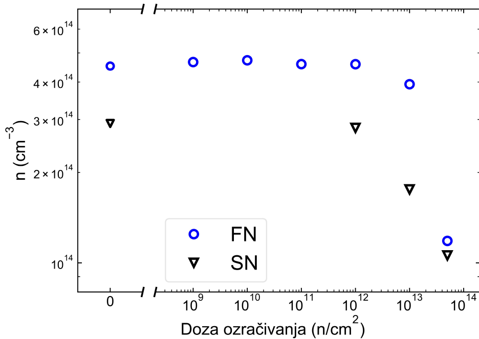
Slika 23. Utjecaj neutronskog ozračivanja na koncentraciju slobodnih nosioca naboja n unutar n-tipa 4H-SiC Schottky dioda. Prikazane vrijednosti su određene regresijom koristeći izraz (4.17) i C-V karakteristike na temperaturi 300 K (Slika 21).
