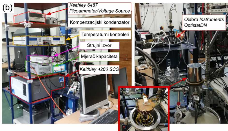
Slika 17. (a) Shema mjernog postava za metode tranzijentne spektroskopije. (b) Položaji komponenti mjernog postava, uključujući Oxford Instruments OptistatDN kriostat te kriostat korišten pri I-V i C-V mjerenjima.
