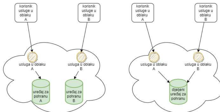
Slika 1.3: Usporedba oblaka bez i sa korištenjem multitenant tehnologije.
