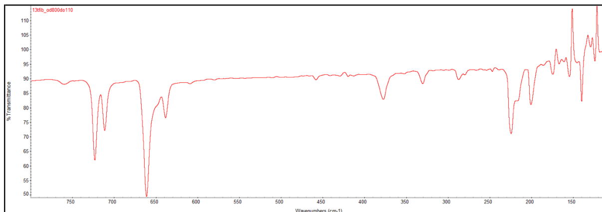
Slika D16. IR spektar spoja 13tfib snimljen tehnikom ATR u području od 800 do 110 \text{cm}^{-1}
