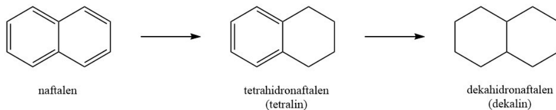
Shema 26. Katalitičko hidrogeniranje naftalena
