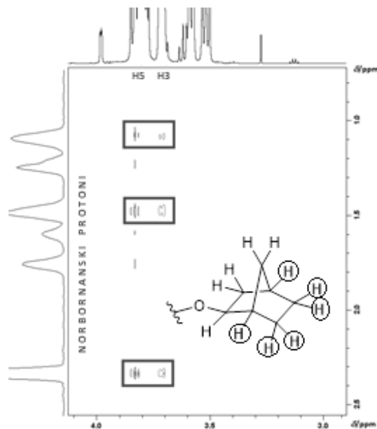
Slika 28. Uvećana regija ROESY spektra kompleksa manokongugata 14 i \beta -ciklodekstrina snimljenog u D_2O pri 25\text{ }^\circ\text{C} s interakcijom kroz prostor, zaokruženi su vodikovi atomi norbornanske podjedinice koji stupaju u interakciju
