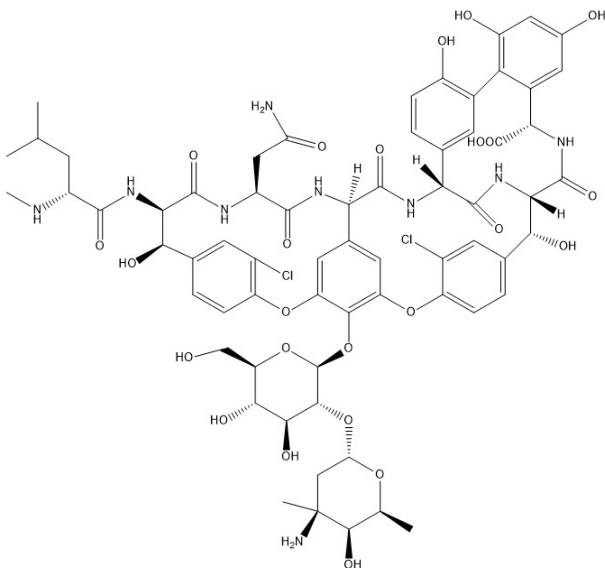
Slika 1. Struktura vankomicina.
