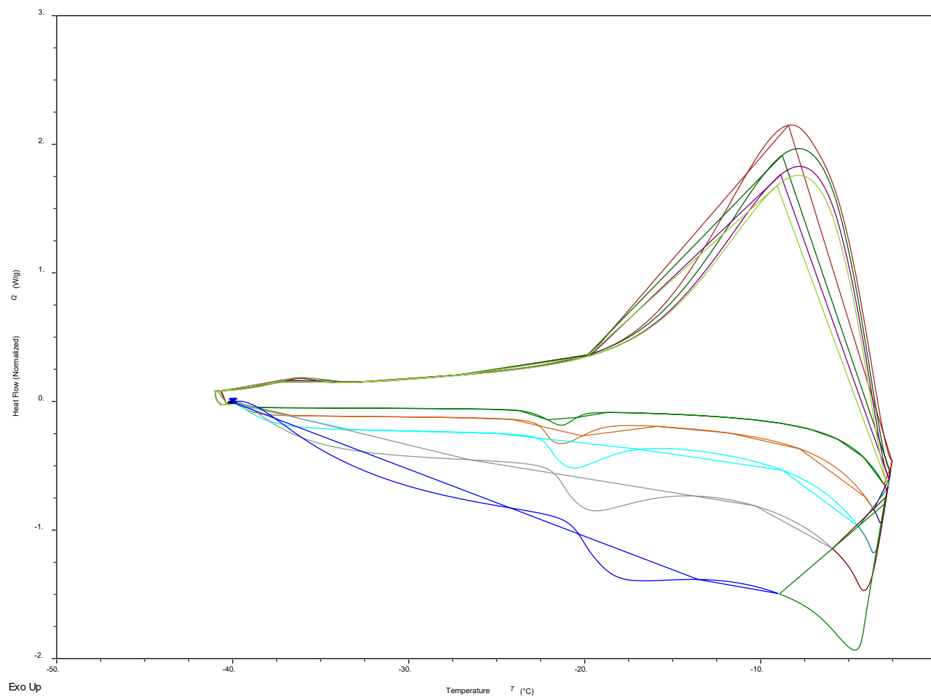
Slika D7A. Ciklička DSC analiza praznih liposoma nakon sonikacije (003S) u rasponu temperatura od -40\text{ }^{\circ}\text{C} do -2\text{ }^{\circ}\text{C} pri različitim brzinama zagrijavanja. Značajan termički prijelaz vidljiv je pri -20\text{ }^{\circ}\text{C} kod zagrijavanja te pri -35\text{ }^{\circ}\text{C} kod hlađenja.
