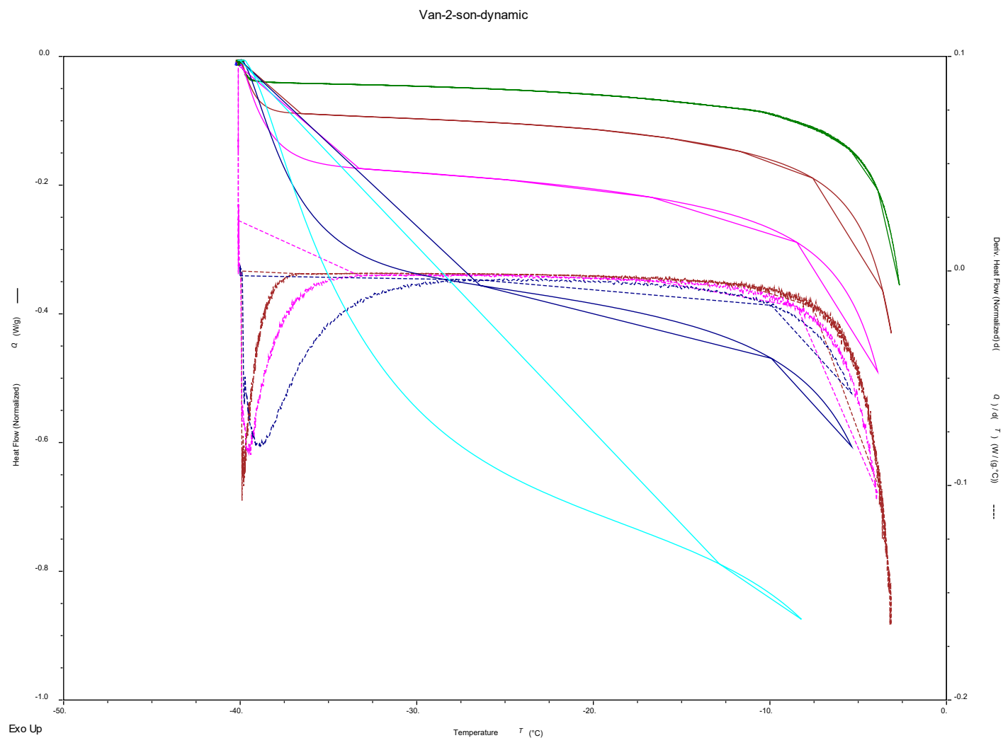
Slika D10B. Ciklička DSC analiza liposoma s vankomicinom nakon sonikacije (002S) u rasponu temperatura od -40\text{ }^\circ\text{C} do -2\text{ }^\circ\text{C} , brzine zagrijavanja gledano od gora prema dolje iznose: 2\text{ }^\circ\text{C}/\text{min} , 5\text{ }^\circ\text{C}/\text{min} , 10\text{ }^\circ\text{C}/\text{min} , 20\text{ }^\circ\text{C}/\text{min} i 40\text{ }^\circ\text{C}/\text{min} . Izostanak maksimuma u 1. derivaciji (iscrtkana krivulja) potvrđuje izostanak termičkih prijelaza u ovom temperaturnom rasponu.
