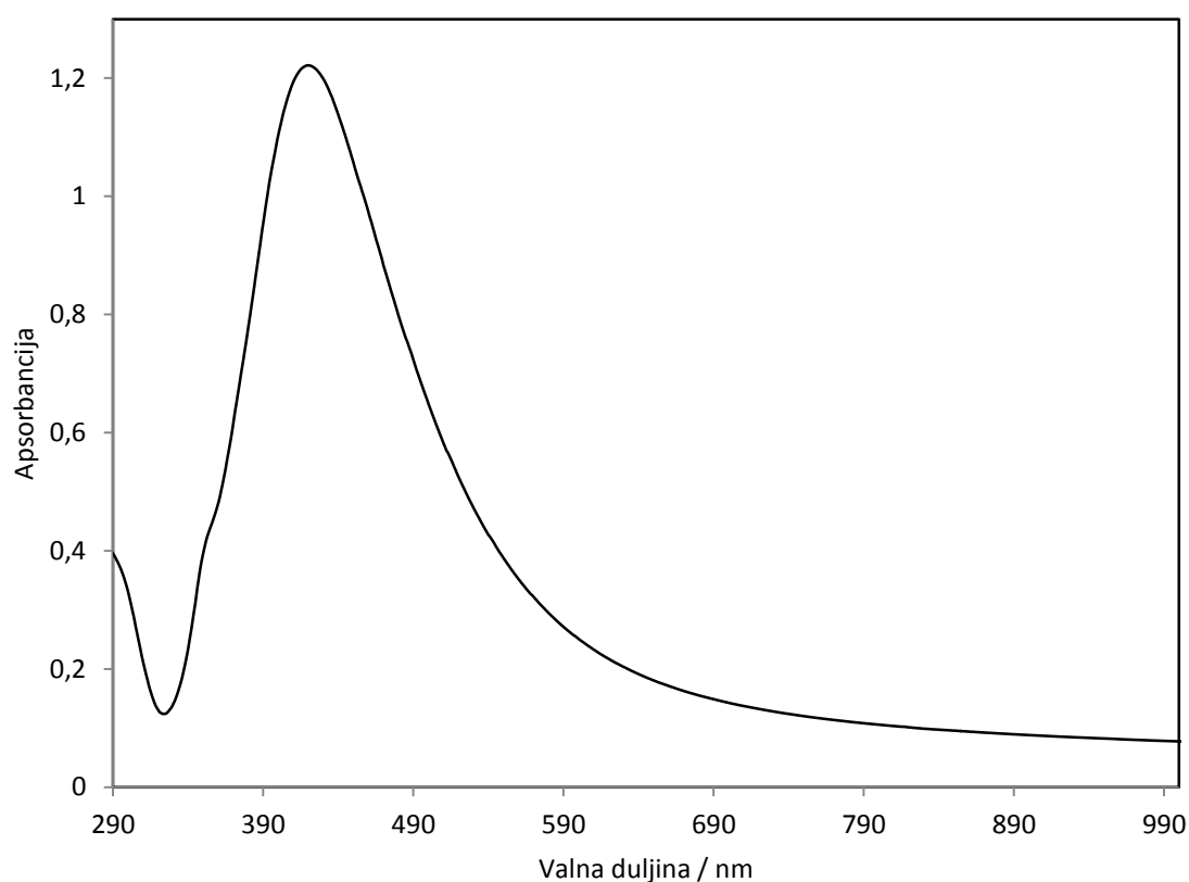
Slika 10. Apsorpcijski spektar koloidne suspenzije srebra
