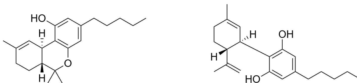
Slika 7. Molekulska struktura Δ-9-THC-a (lijevo) i CBD-a (desno). Slika je izrađena pomoću ChemDraw Direct-a . 26
