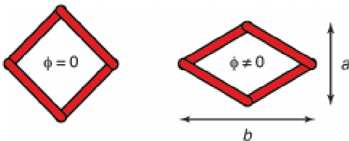
Slika 3. Paraelastično (lijevo) i feroelastično (desno) stanje kvadratne rešetke. Feroelastični parametar \phi = (b - a) / (a + b) mjera je za razmjer izobličenja koje narušava simetriju kvadratne rešetke.
