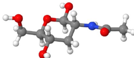
(b) N-acetil-D-glukozamin. Slika preuzeta od: "Kevinjh, CC BY-SA 3.0, via Wikimedia Commons"
