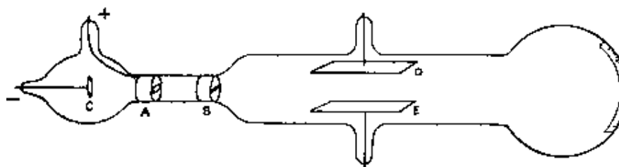
Slika 1.3: Thomsonov eksperiment [15]
