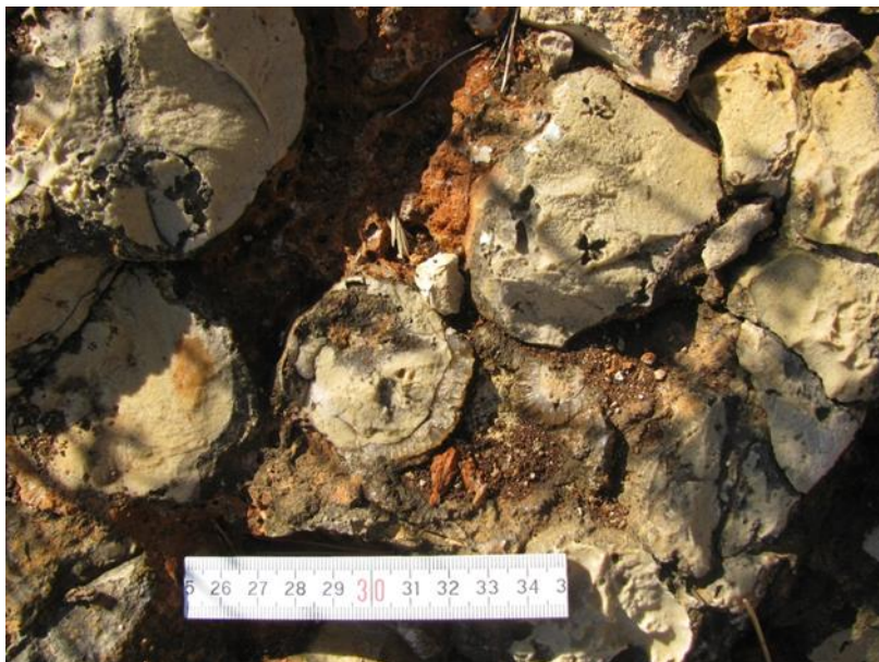
Slika 24 Krupniji „prstasti“ ostaci koralja na gornjoj slojnoj površini grebena 8 (mjerilo je dužine 10 cm).
