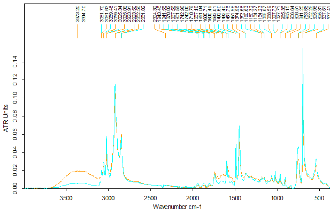
Slika 38. Usporedba spektara Interne baze 6b (narančasta) i Interne baze 6b H 2 O 2 (svijetlo plava)
