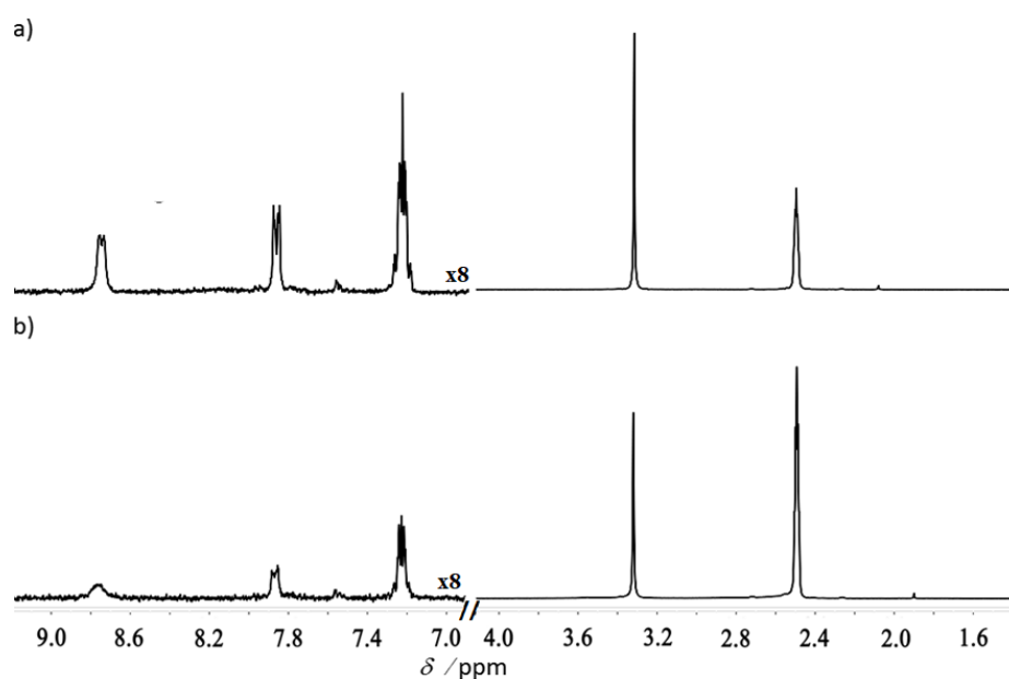
Slika 8.39: Aromatski dio ( lijevo ) i alifatski dio ( desno ) ^1\text{H-NMR} spektara produkta D1-IIIb dobivenog reakcijom izmjene korištenjem LiCl iz a) D1-IIa b) D1-Id . Spektri su snimljeni u \text{DMSO-}d_6 .
