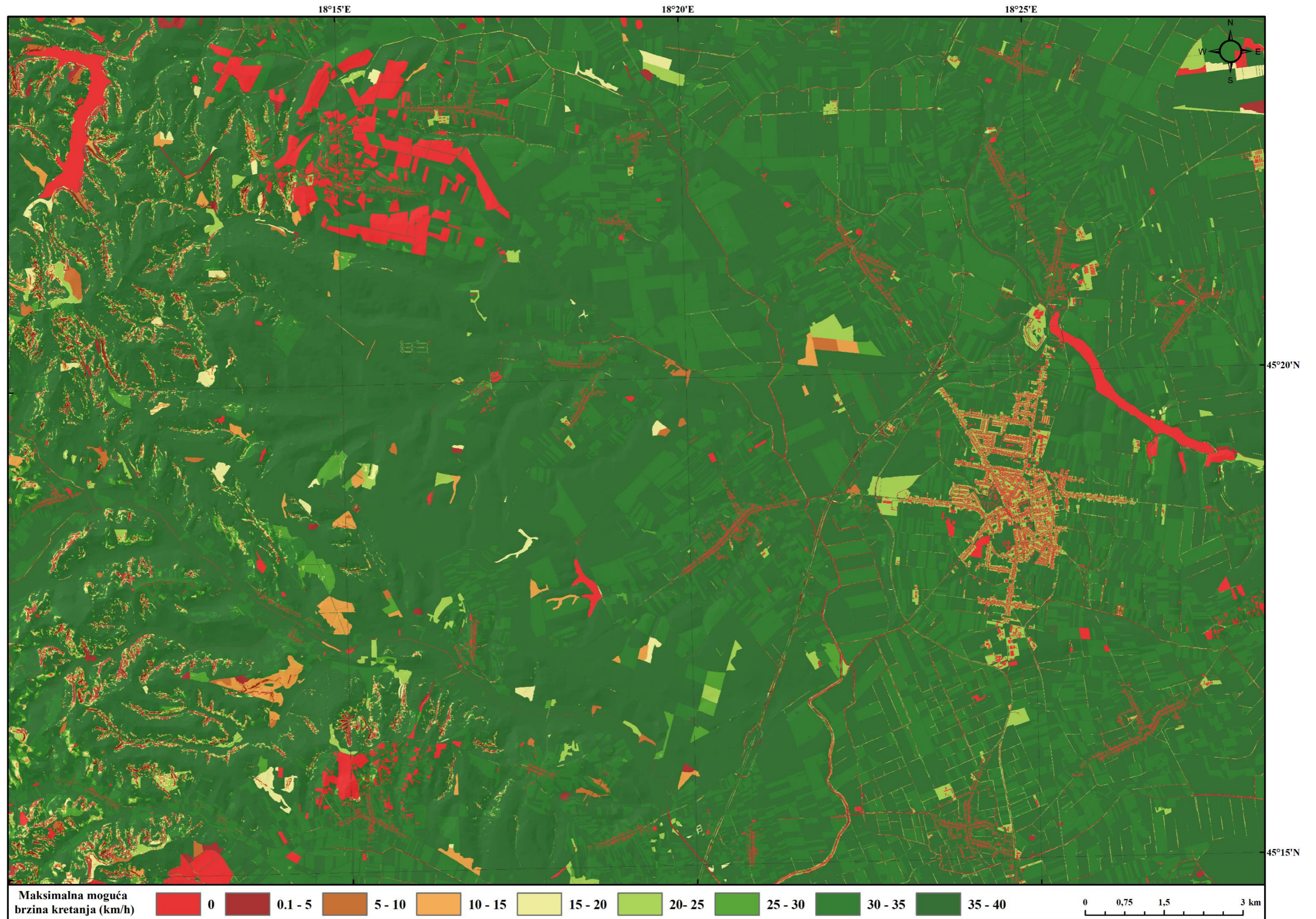
Sl. 93. Karta maksimalne brzine kretanja za BTR-50 (ljet/jesen – suho)
