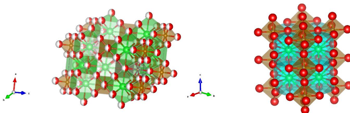
Slika 41. Struktura heksagonskog Ba 3 Fe 2 WO 9 (lijevo) i tetragonskog Sr 3 Fe 2 WO 9 (desno).
