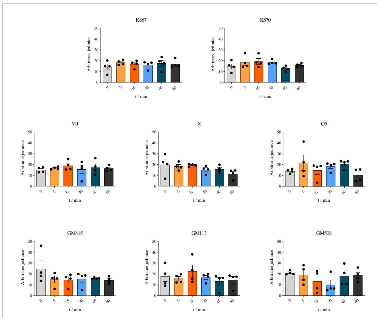
Slika 4.10. Fosforilacija NF-κB nakon 5 – 60 min tretmana SH-SY5Y stanica odabranim oksimima: K870 (15 μmol dm -3 ), K867 (400 μmol dm -3 ), X (200 μmol dm -3 ), VII (250 μmol dm -3 ), Q5 (100 μmol dm -3 ), GM415 (350 μmol dm -3 ), GM113 (300 μmol dm -3 ), GM508 (50 μmol dm -3 ). Vrijednosti su prikazane kao srednja vrijednost eksperimentalno dobivenih vrijednosti (± standardna pogreška). Parametri su evaluirani iz najmanje četiri pokusa.
