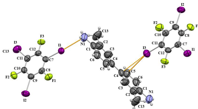
Slika 48. ORTEP prikaz jedinice kokristala (otol)(135tfib) 2 . Svi atomi su prikazani elipsoidima pomaka s 50% vjerojatnošću. Atomi vodika su prikazani kuglicama veličine 0,15 Å. Halogenske veze I \cdots N te I \cdots \pi prikazane su narančastim isprekidanim crtama
