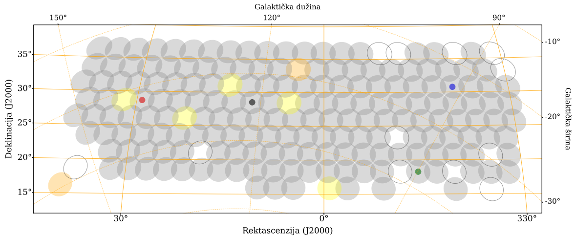
Slika 2.2. Polja od kojih je napravljen mozaik u projekciji na ekvatorijalni koordinatni sustav, galaktička koordinatna mreža je označena isprekidanim linijama. Veličine krugova odgovaraju maksimalnoj veličini primarnog odgovora teleskopa koja iznosi 4.74^\circ . Opažanja u poljima označenim sivim krugovima su u rasponu frekvencija 120 – 167 MHz, žutim krugovima u rasponu 120 – 165 MHz i narančastim krugovima u rasponu 120 – 163 MHz. Sive kružnice označavaju polja koja su izbačena iz izrade mozaika zbog prevelikog šuma. Točkama su označena polja čiji su grafovi šuma prikazan na slici 2.3., boje točaka odgovaraju boji grafova.
