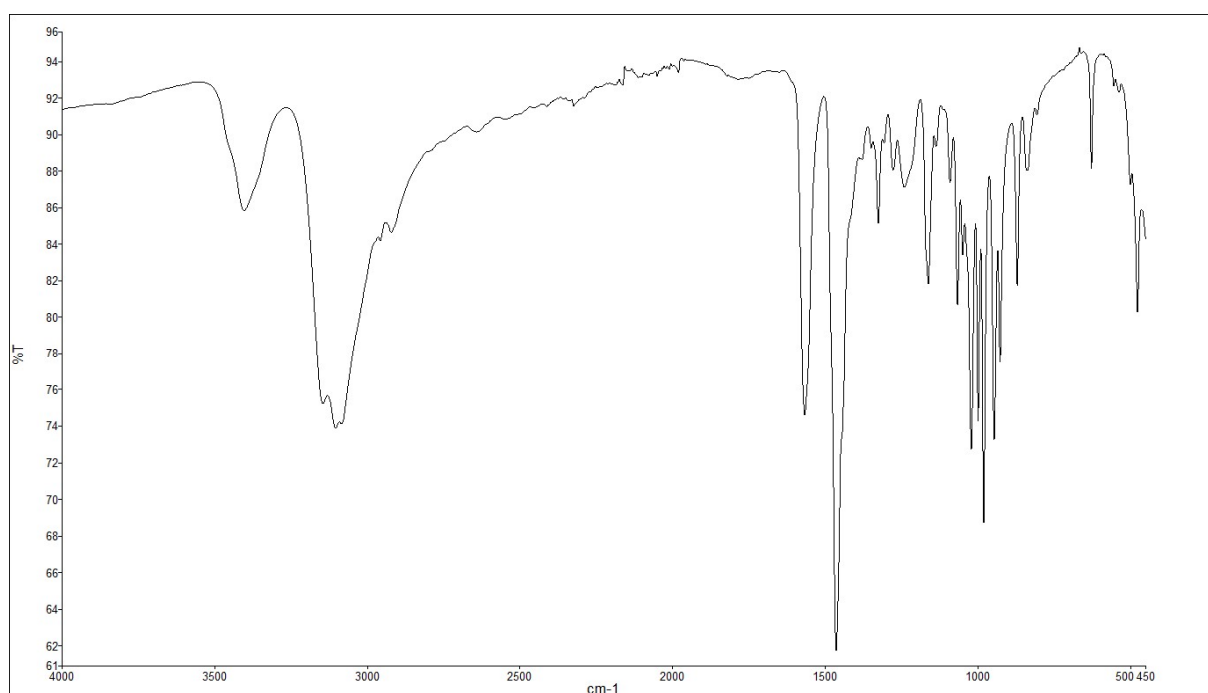
Slika D18. IR spektar \text{H}_2(\text{DPOH})[\text{CuBr}_4] . Spoj je dobiven mehanokemijskom sintezom uz etanol kao tekućinu kojom je bilo potpomognuto mljevenje
