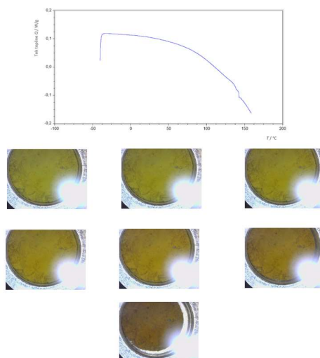
Slika D36. DSC krivulja spoja \text{H}_2(\text{DPOH})[\text{CuCl}_4] . Ispod su prikazane fotografije istog spoja snimljene pri -39,58\text{ }^\circ\text{C} , 0,13\text{ }^\circ\text{C} , 40,15\text{ }^\circ\text{C} , 80,15\text{ }^\circ\text{C} , 120,14\text{ }^\circ\text{C} , 140,12\text{ }^\circ\text{C} , 158,43\text{ }^\circ\text{C} .
