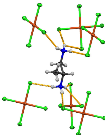
Slika 27. Prikaz vodikovih veza uzorka \text{H}_2(1,2\text{-DAP})[\text{CuCl}_4] . Elipsoidi pomaka nevodikovih atoma prikazani su s vjerojatnošću 30 %, a vodikovi atomi su prikazani kao kuglice proizvoljnog radijusa. Vodikove veze istaknute su zelenom isprekidanom linijom
