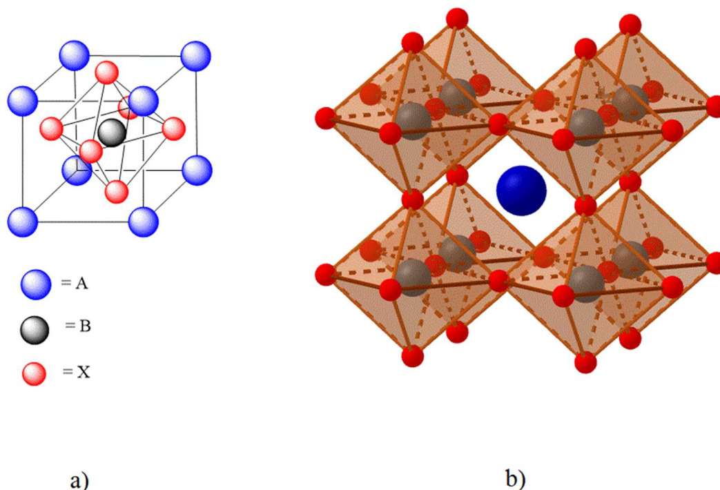
Slika 2. Struktura halogenidnog perovskita formule ABX_3 (A = jednovalentni kation; B = divalentni kation poput Pb^{2+} , Ge^{2+} , Sn^{2+} ; X = Cl^- , Br^- ili I^- )
