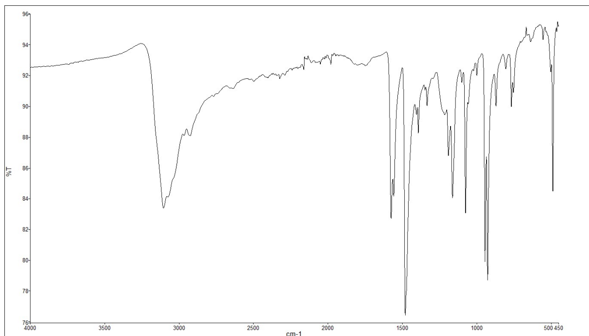
Slika D23. IR spektar \text{H}_2(1,3\text{-DAP})[\text{CuBr}_4] . Spoj je dobiven mehanokemijskom sintezom uz acetonitril kao tekućinu kojom je bilo potpomognuto mljevenje
