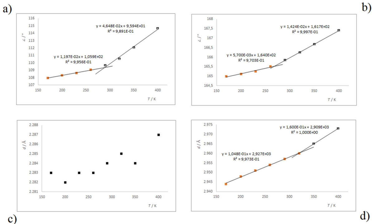
Slika 30. Grafički prikazi \Delta(3C \text{ atoma}) (a), \Delta(Cu-Cl_{ekv}-Cu) (b), d(Cu-Cl_{ekv})_s (c), d(Cu-Cl_{ekv})_l (d) u ovisnosti o temperaturi za spoj H_2(1,3-DAP)[CuCl_4] . Sjecišta na grafičkim prikazima su pri temperaturama 289 K (a), 269 K (b) i 326 K (d)
