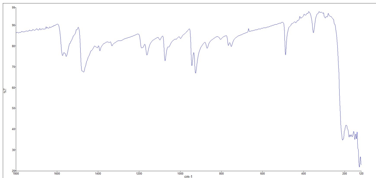
Slika D28. Far-IR spektar \text{H}_2(1,3\text{-DAP})[\text{CuBr}_4] . Spoj je dobiven otopinskom sintezom uz acetonitril kao otapalo
