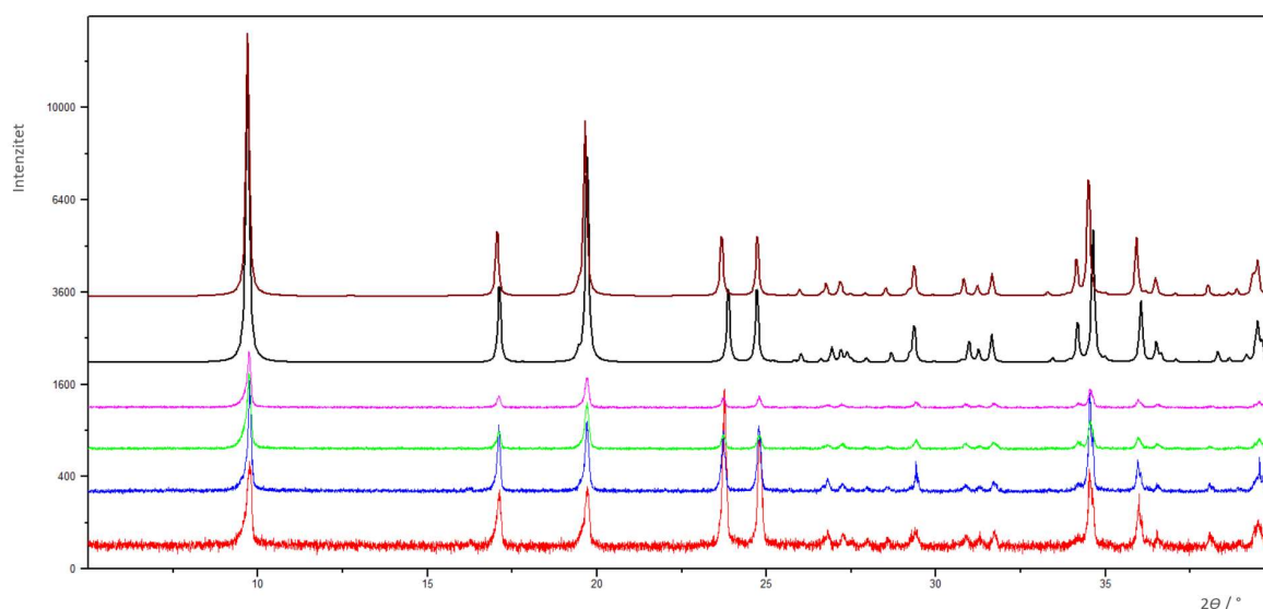
Slika D35. Difraktogrami praškastih uzoraka \text{H}_2(1,3\text{-DAP})[\text{CuCl}_4] . Crveni odnosno plavi difraktogram predstavlja uzorak \text{H}_2(1,3\text{-DAP})[\text{CuCl}_4] dobiven otopinskom sintezom uz acetonitril odnosno etanol kao otapalo. Zeleni odnosno ljubičasti difraktogram predstavlja isti spoj dobiven mehanokemijskom sintezom koristeći acetonitril odnosno etanol kao tekućinu kojom je bilo potpomognuto mljevenje. Crni predstavlja izračunati difraktogram praha iz literaturno određene strukture spoja \text{H}_2(1,3\text{-DAP})[\text{CuCl}_4] , a smeđi predstavlja izračunati difraktogram praha iz strukture spoja \text{H}_2(1,3\text{-DAP})[\text{CuCl}_4] koja je određena pri 290 K u okviru izrade ovog diplomskog rada
