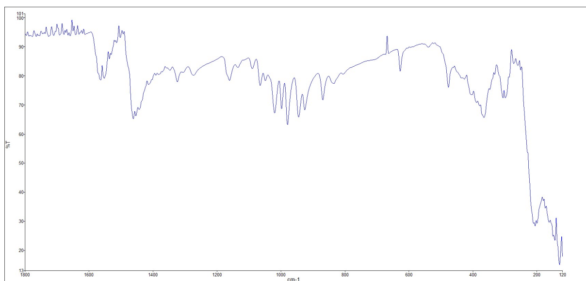
Slika D24. Far-IR spektar \text{H}_2(\text{DPOH})[\text{CuBr}_4] . Spoj je dobiven otopinskom sintezom uz acetonitril kao otapalo
