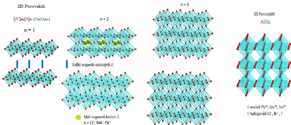
Slika 3. Shematski prikaz HOAH slojevitih struktura (2D perovskiti) i shematski prikaz strukture trodimenzijskih perovskita s kojom su slojeviti HOAH strukturno povezani
