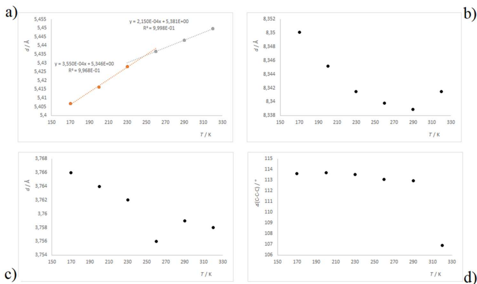
Slika 35. Grafički prikazi a) d(\text{Cu—Cu})_{\text{ip}} , b) d(\text{Cu—Cu})_{\text{oop}} , c) d(\text{N—N}) , d) \angle(\text{3C atoma}) u ovisnosti o temperaturi za spoj \text{H}_2(1,2\text{-DAP})[\text{CuCl}_4] . Sjecište se nalazi na temperaturi od: a) 250 K
