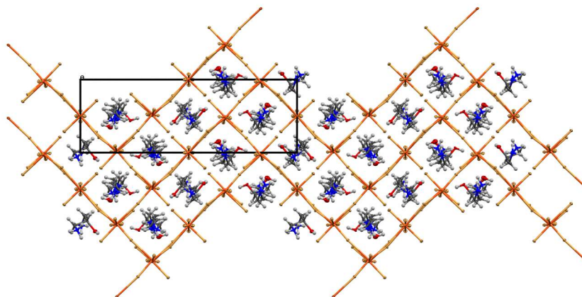
Slika 14. Prikaz pakiranja H_2(DPOH)[CuBr_4] duž a smjera. Elipsoidi pomaka nevodikovih atoma prikazani su s vjerojatnošću 30 %, a vodikovi atomi su prikazani kao kuglice proizvoljnog radijusa
