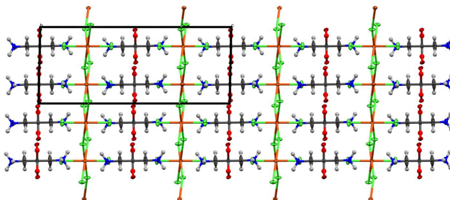
Slika 8. Prikaz pakiranja \text{H}_2(\text{DPOH})[\text{CuCl}_4] duž b smjera. Elipsoidi pomaka nevodikovih atoma prikazani su s vjerojatnošću 30 %, a vodikovi atomi su prikazani kao kuglice proizvoljnog radijusa
