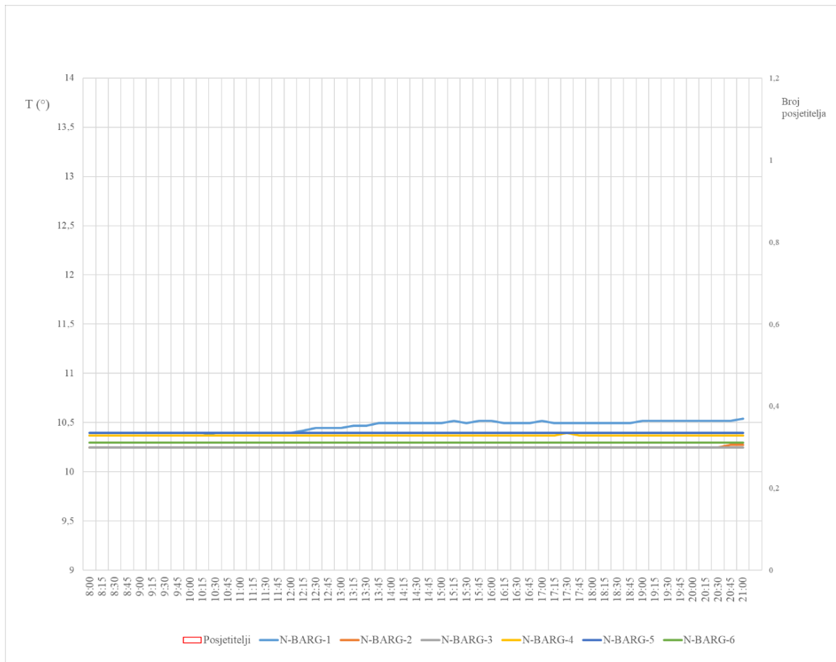
Slika 25 – Kretanje trenutnih vrijednosti temperature zraka na svim mjernim postajama na dan 2. studenog 2019. bez posjetitelja
