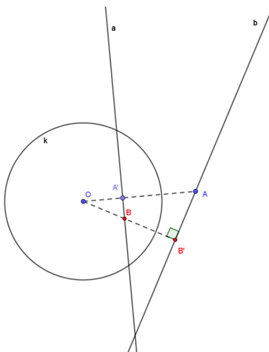
Slika 2.9: Skica leme 2.1.9.
