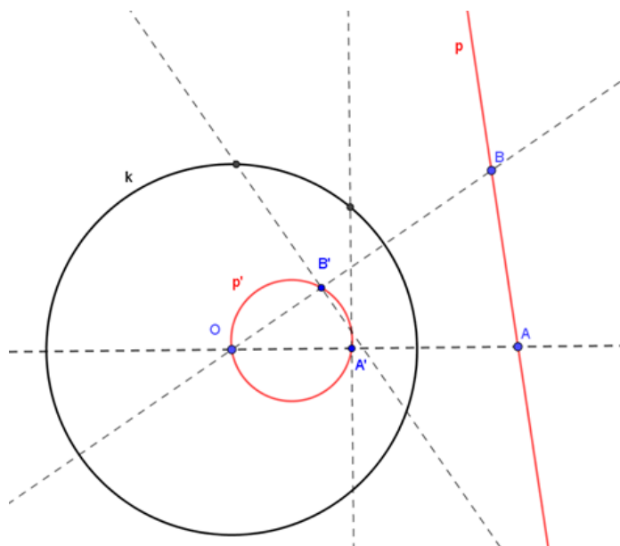
Slika 1.10: Inverzna slika pravca p koji ne prolazi kroz središte inverzije O
