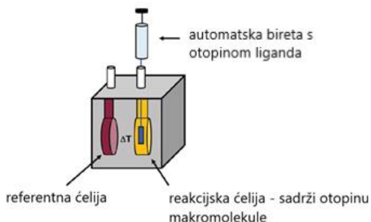
Slika 12. Shematski prikaz izoternnog titracijskog kalorimetra. 39 autom bireta
