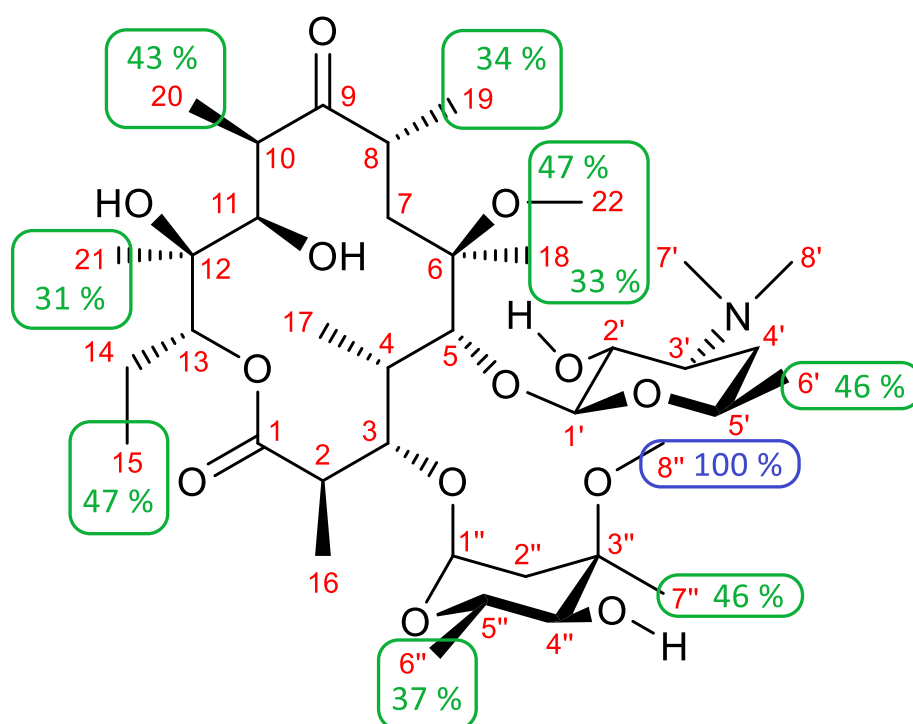
Slika 39. Epitopi vezanja klaritromicina u \text{D}_2\text{O} izračunati iz spektara STD.
