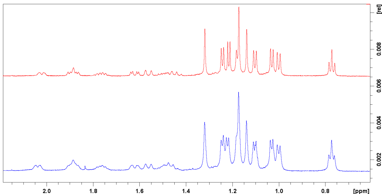
Slika 34. Uvećani prikaz dijela spektra (0–2,0 ppm) ^1\text{H} NMR klaritromicina u \text{D}_2\text{O} prije (crveno) i nakon dodatka ribosoma (plavo).
