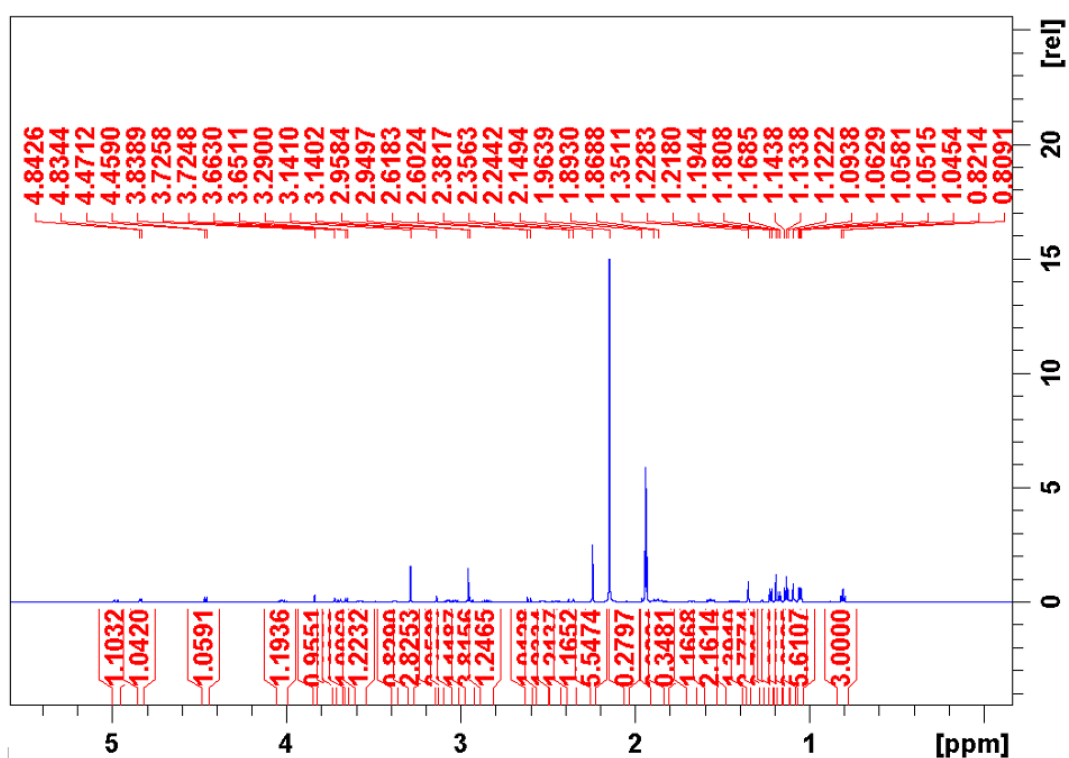
Slika D6. Spektar 1 H NMR klaritromicina u acetonitrilu-d 3 .
