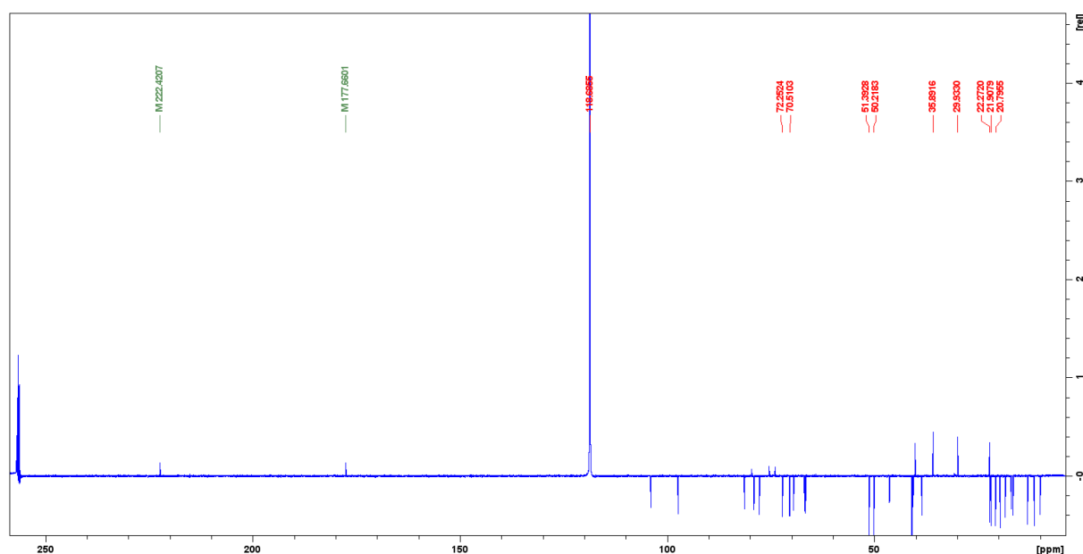
Slika D7. Spektar DEPT-Q klaritromicina u acetonitrilu-d 3 .
