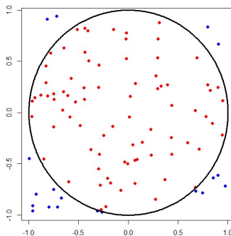
Slika 4.1: Grafički prikaz simuliranog uzorka duljine n = 10^2
