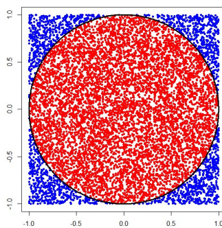
Slika 4.2: Grafički prikaz simuliranog uzorka duljine n = 10^4
