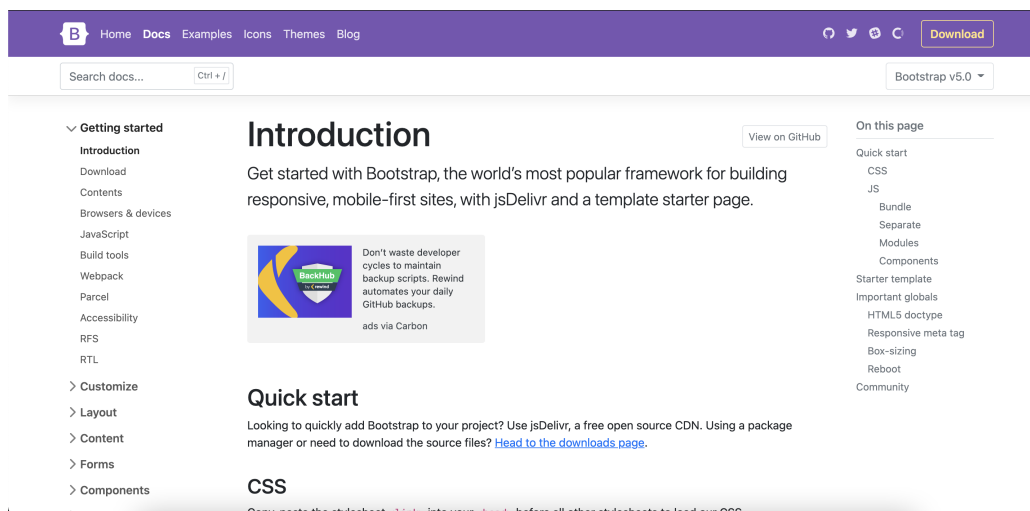
Slika 3.23: Dokumentacija Bootstrap-a
